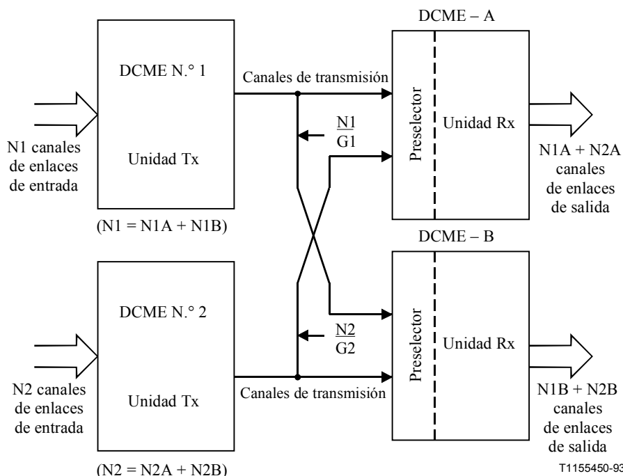
Figura 4/Q.50 – Modo multidestino (sólo se indica un sentido de transmisión)
