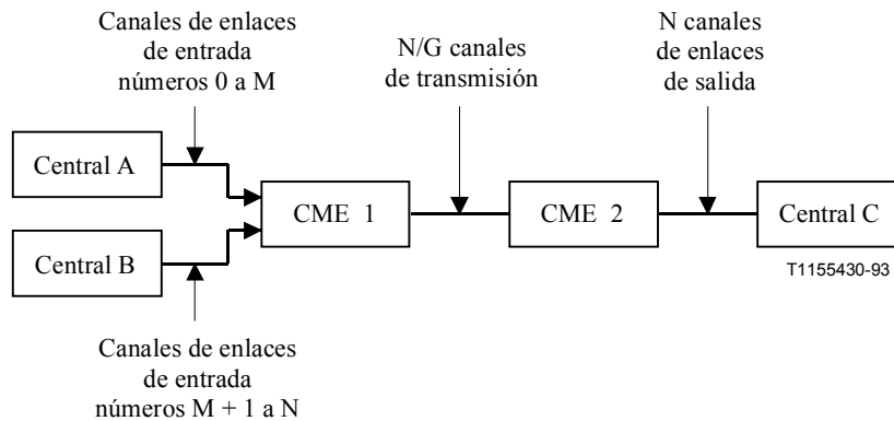
b) Punto a punto unidireccional con dos orígenes
