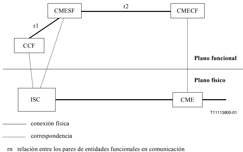
Figura 5/Q.50 – Modelo conceptual de la metodología utilizada
