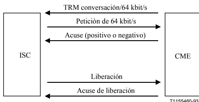
Figura 6/Q.50 – Flujos de información típicos entre el centro de conmutación internacional y el equipo de multiplicación de circuitos
