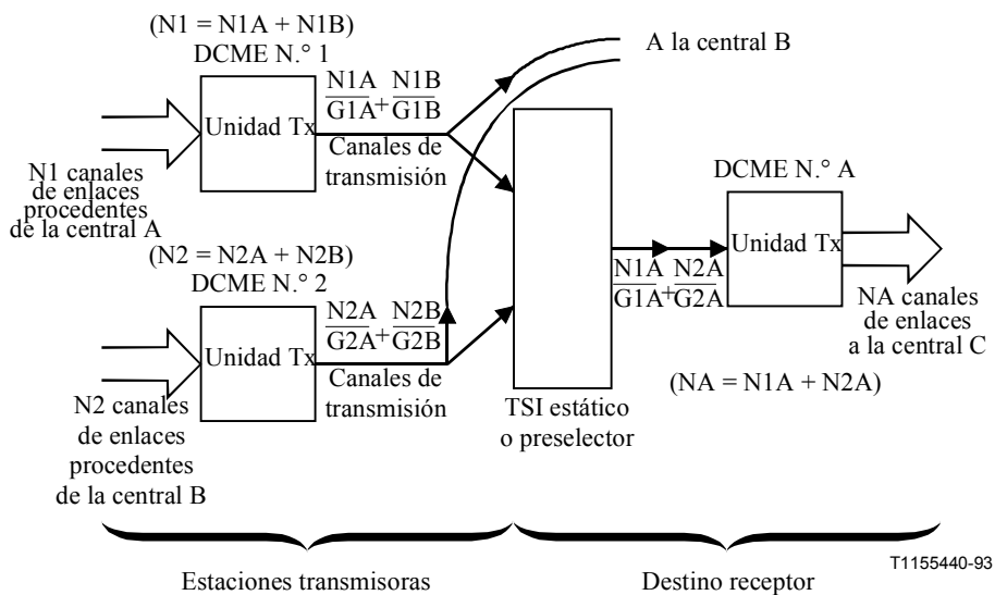
Figura 3/Q.50 – Modo multiasociación (sólo se indica un sentido de transmisión)
