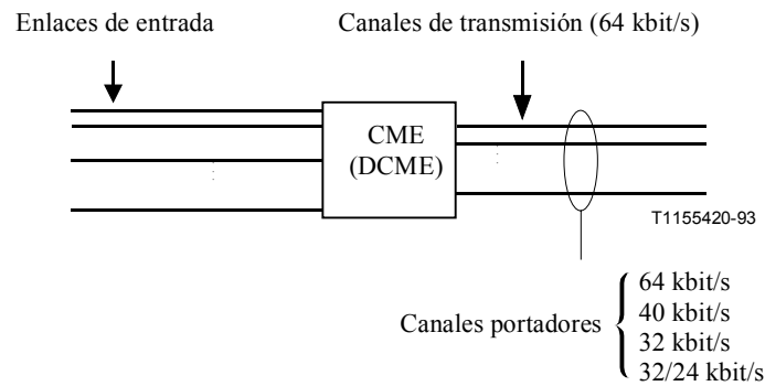
Figura 1/Q.50 – Ganancia del equipo de multiplicación de circuitos
