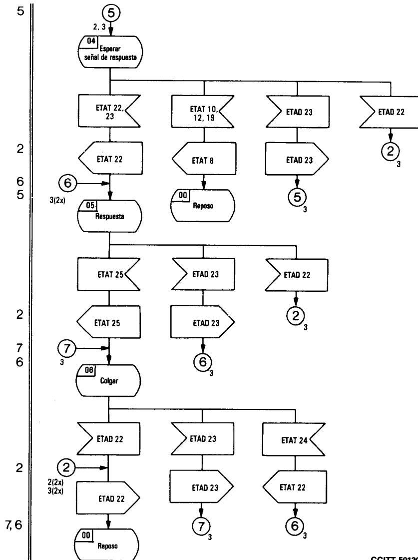
FIGURA 3/Q.642 (hoja 3 de 3) Interfuncionamiento del sistema de señalización N.º 5 hacia el N.º 6
