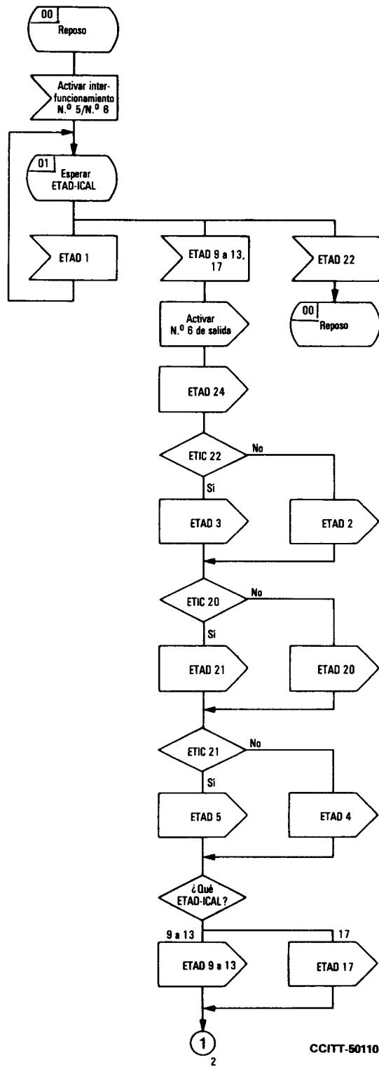
FIGURA 3/Q.642 (hoja 1 de 3) Interfuncionamiento del sistema de señalización N.º 5 hacia el N.º 6
