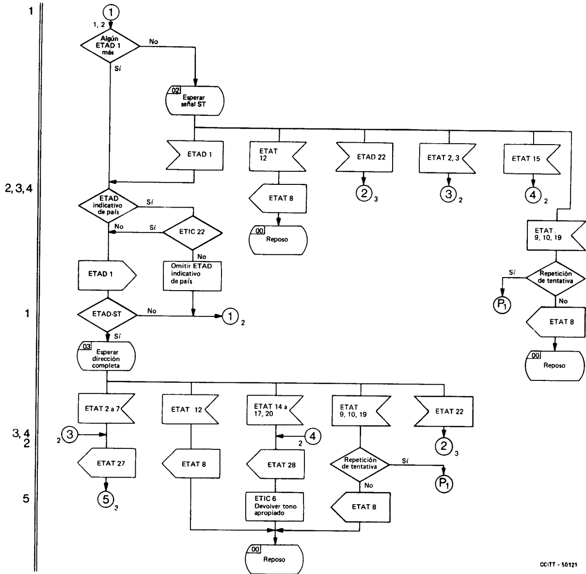
FIGURA 3/Q.642 (hoja 2 de 3)
