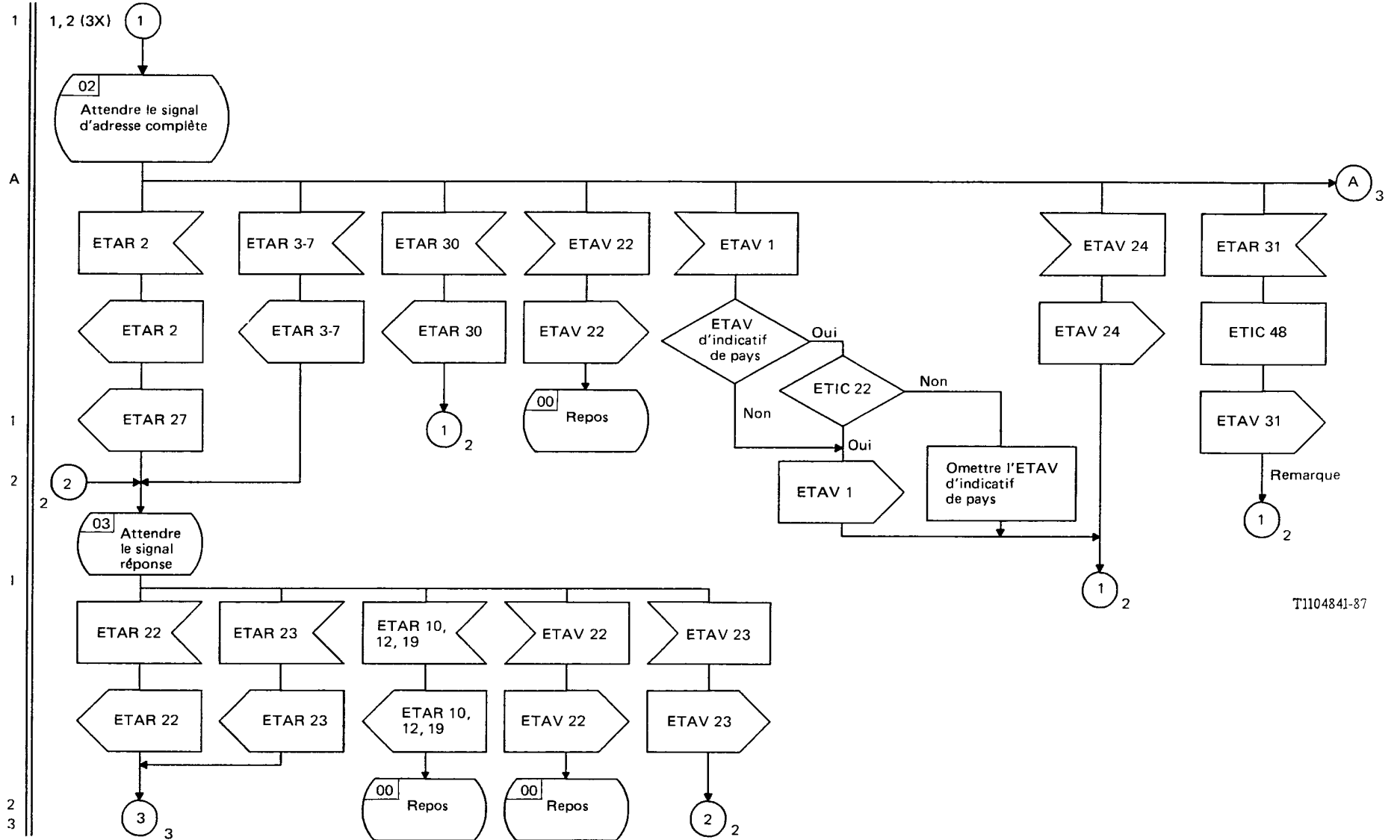
FIGURE 3/Q.653 (feuillet 2 sur 3) Interfonctionnement n° 6 vers n° 7 (SSUT)
