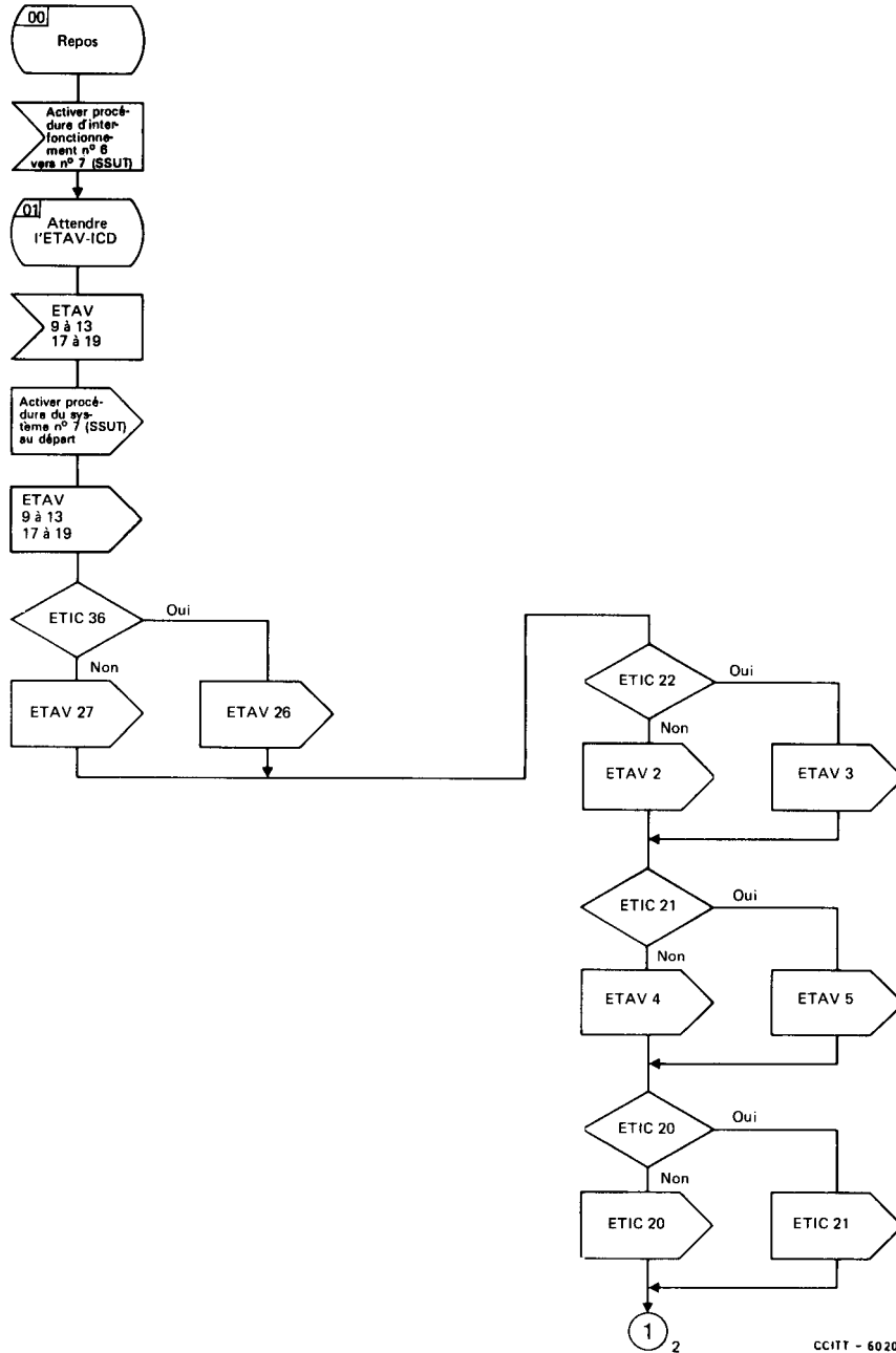
FIGURE 3/Q.653 (feuillet 1 sur 3)
