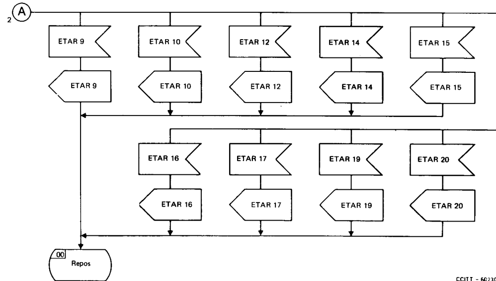
FIGURE 3/Q.653 (feuillet 3 sur 3)
