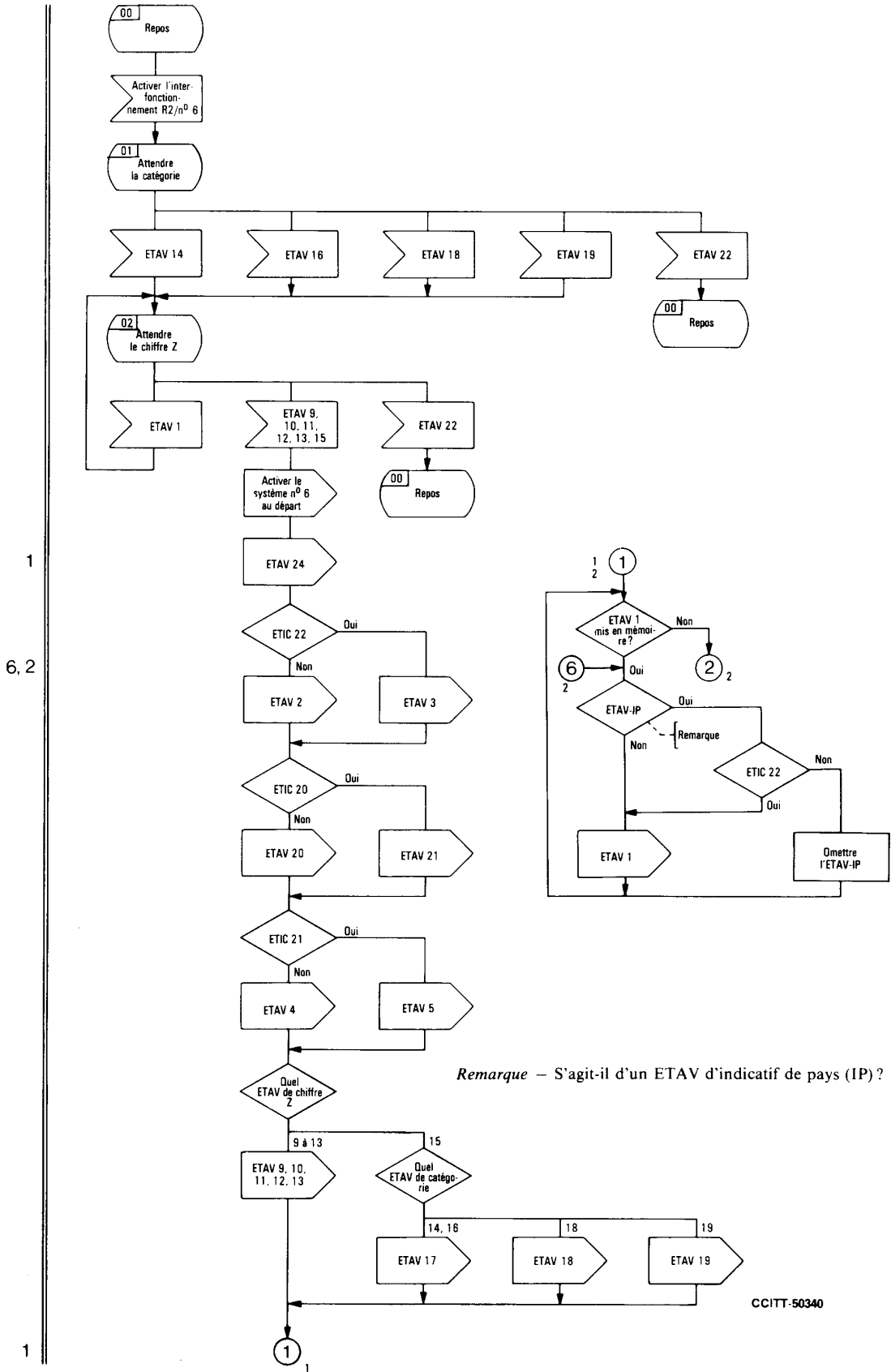
FIGURE 3/Q.683 (feuillet 1 sur 2) Interfonctionnement R2 vers n° 6
