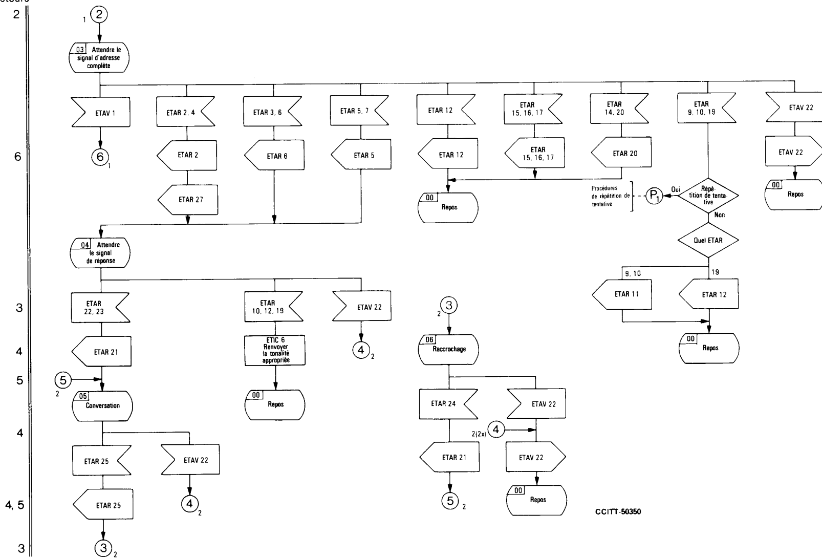
FIGURE 3/Q.683 (feuillet 2 sur 2) Interfonctionnement R2 vers n° 6
