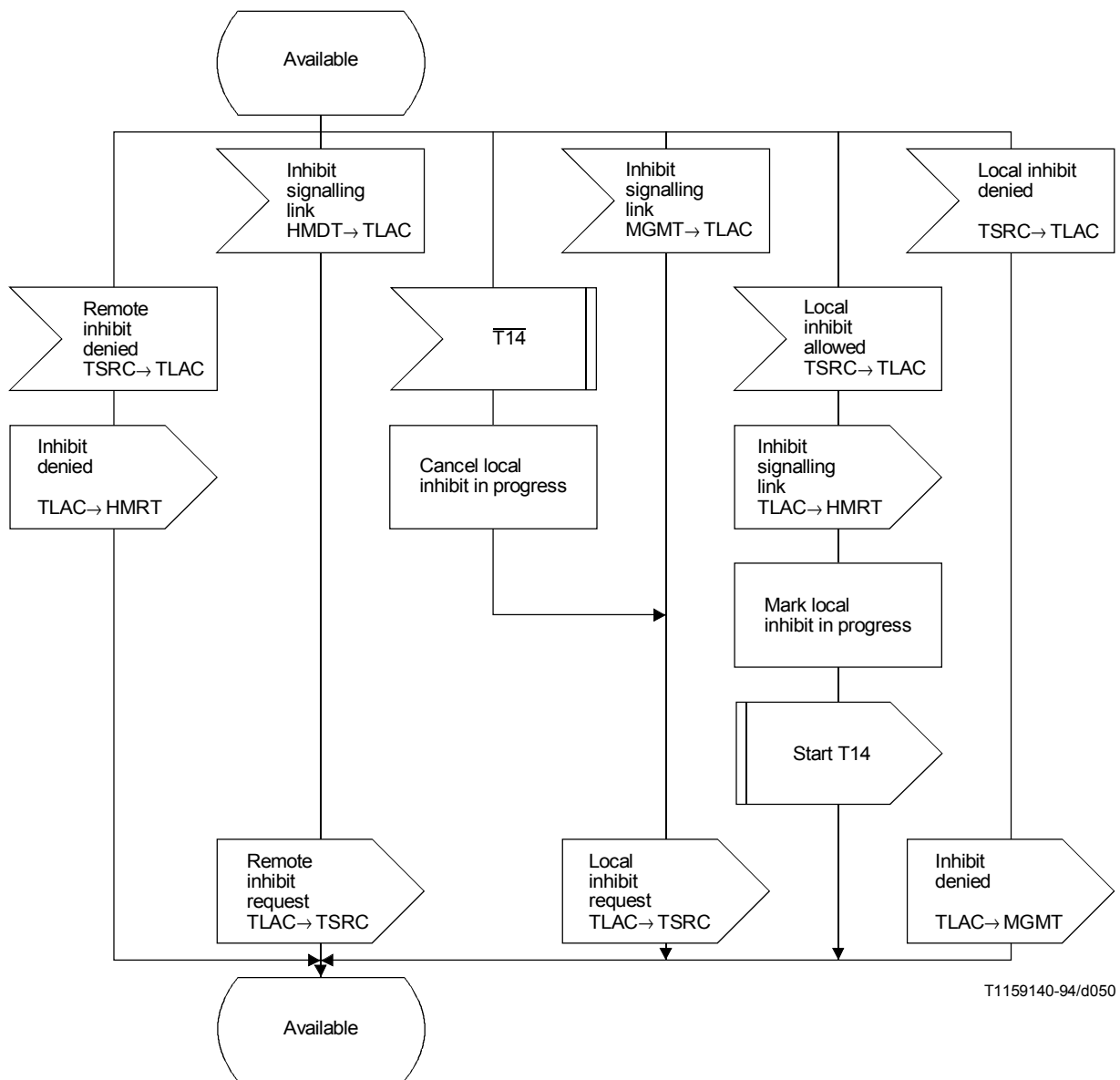
FIGURE 28/Q.704 (feuillet 1 sur 18) Gestion du trafic sémaphore; contrôle de la disponibilité des canaux sémaphores (TLAC)
