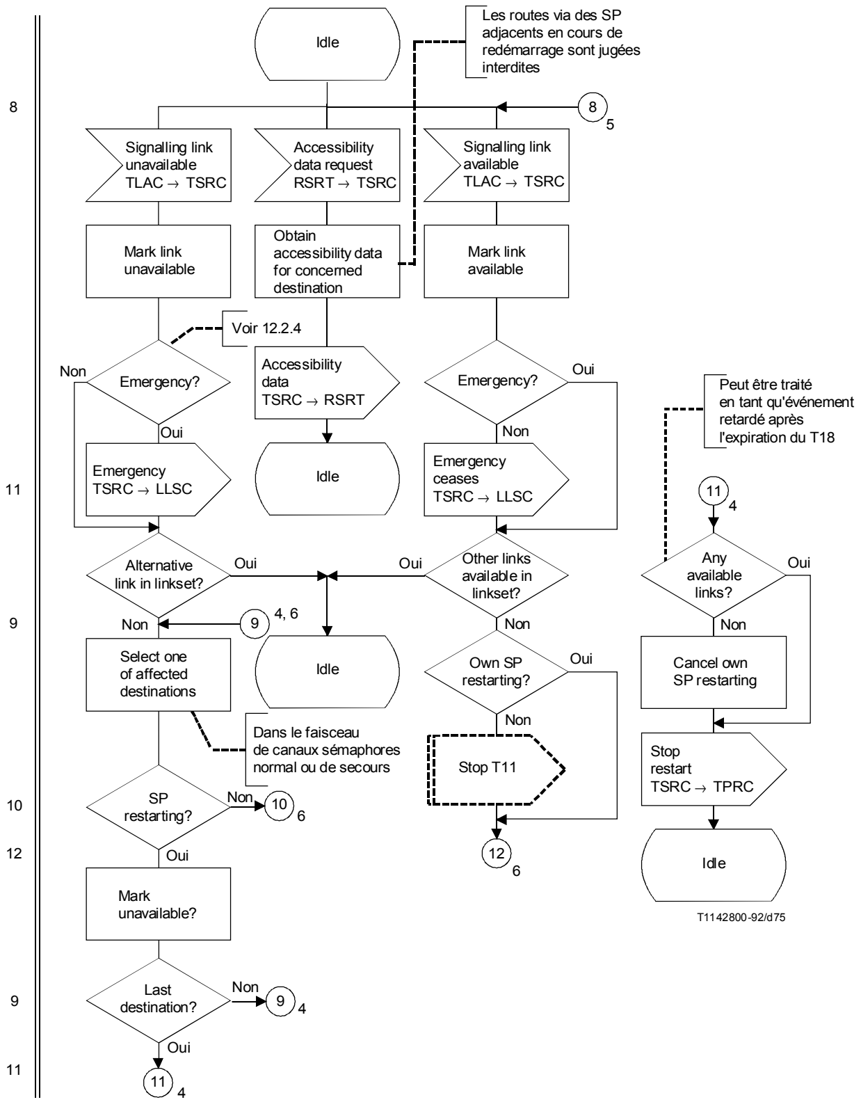
FIGURE 29/Q.704 (feuille 4 sur 21)
