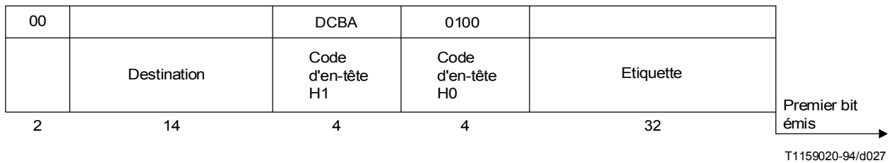
FIGURE 18/Q.704 Message d'interdiction de transfert
