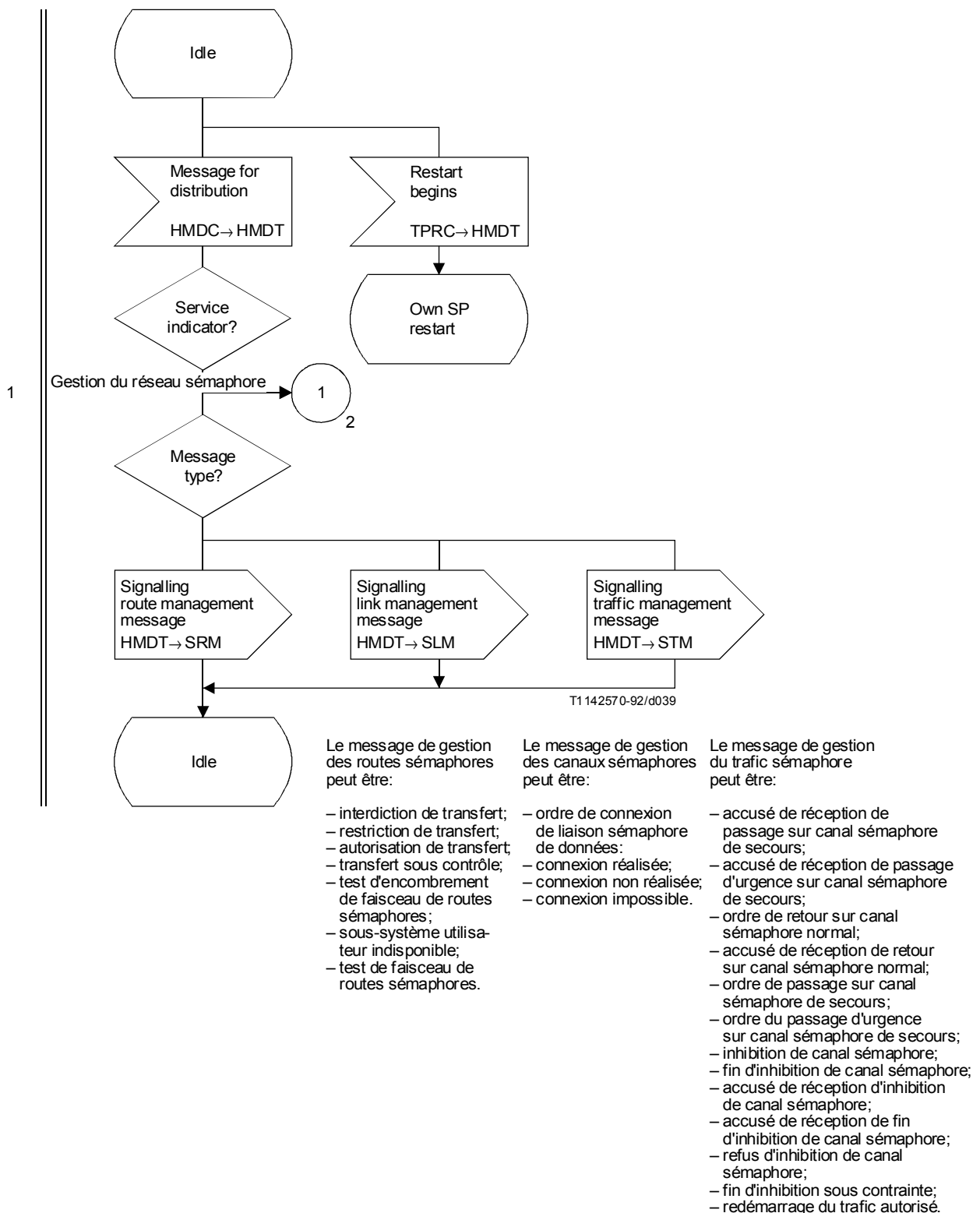
FIGURE 25/Q.704 (feuillet 1 sur 3) Orientation des messages de signalisation; distribution des messages (HMDT)
