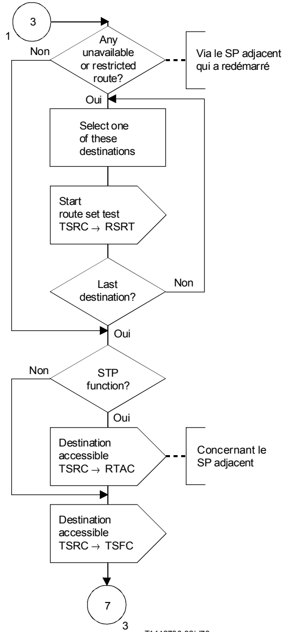
FIGURE 29/Q.704 (feuillet 2 sur 21)
