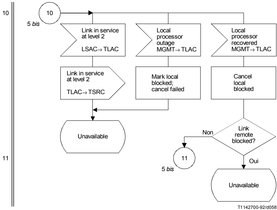
FIGURE 28/Q.704 (feuillet 6 bis sur 18)
