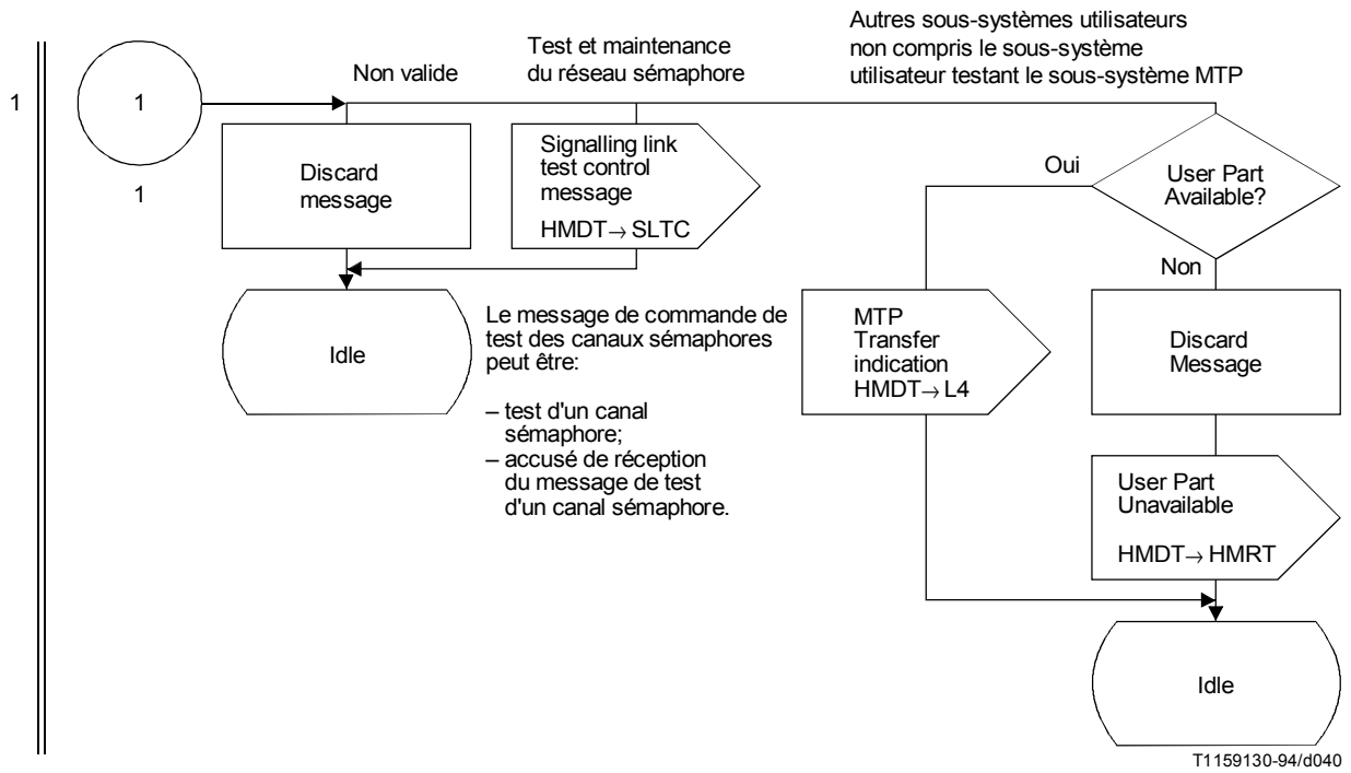
FIGURE 25/Q.704 (feuillet 2 sur 3)
