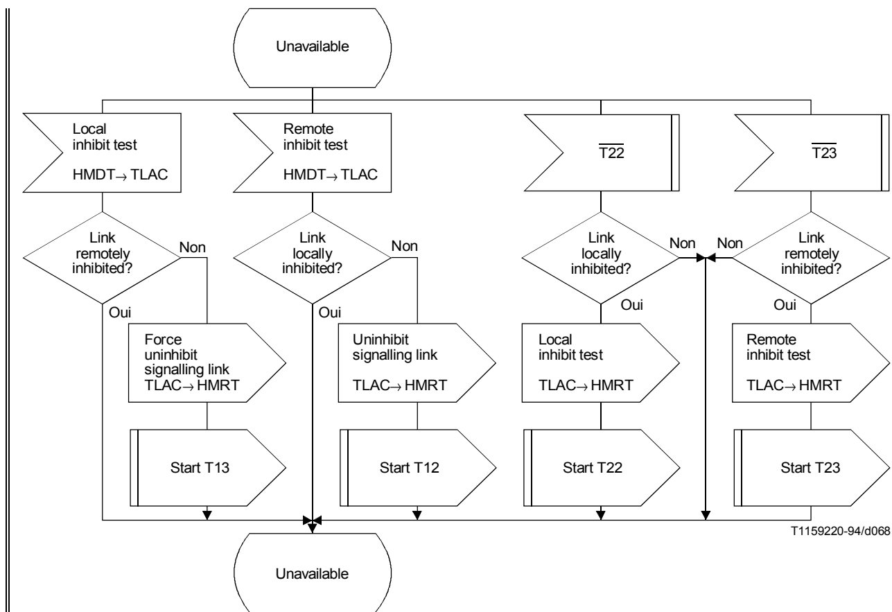
FIGURE 28/Q.704 (feuillet 15 sur 18) Gestion du trafic sémaphore; contrôle de la disponibilité des canaux sémaphores (TLAC)
