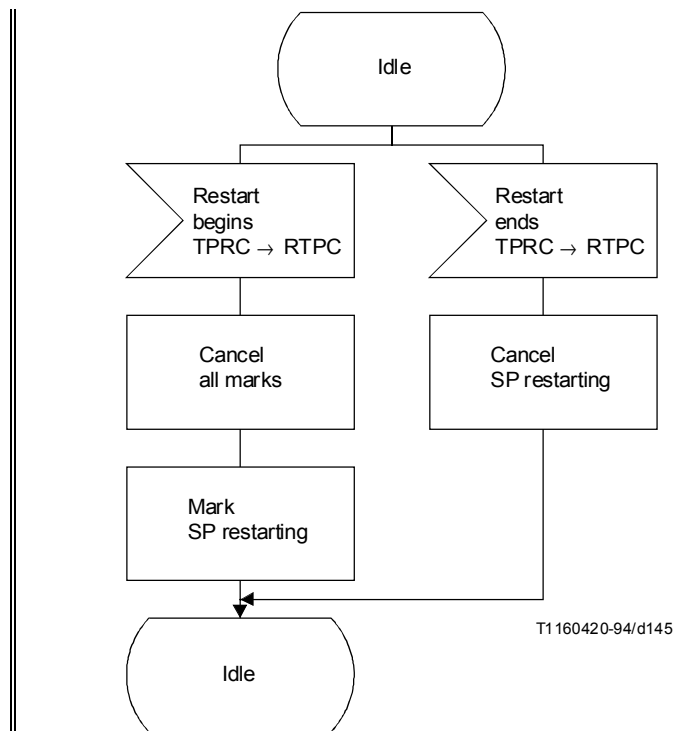
FIGURE 44/Q.704 (feuillet 3 sur 3) Gestion des routes sémaphores; commande d'interdiction de transfert (RTPC)
