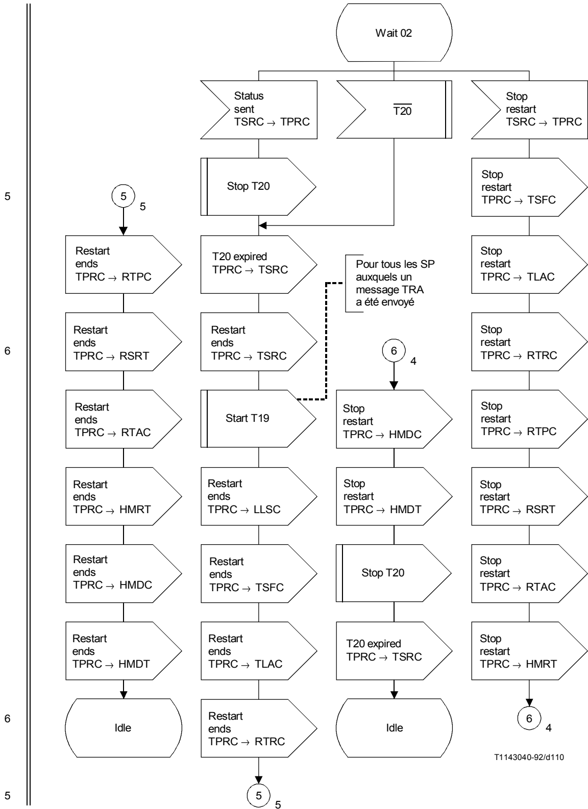
FIGURE 34b/Q.704 (feuillet 5 sur 7)
