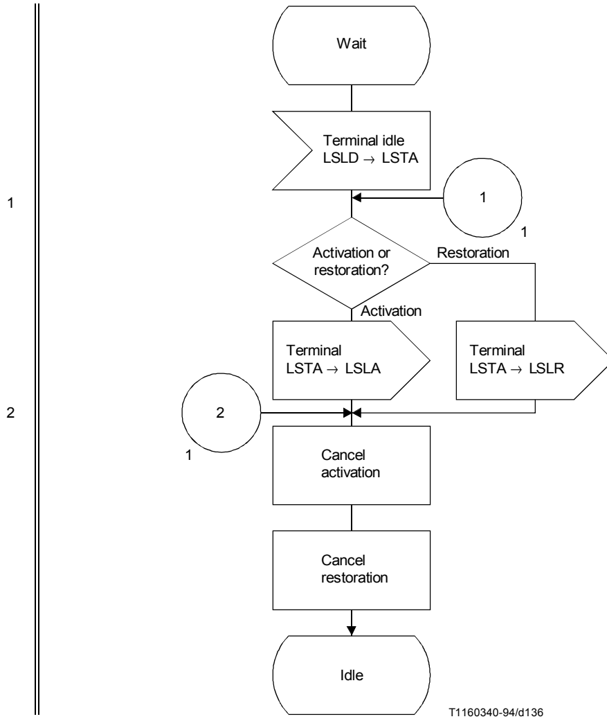
FIGURE 41/Q.704 (feuillet 2 sur 2)
