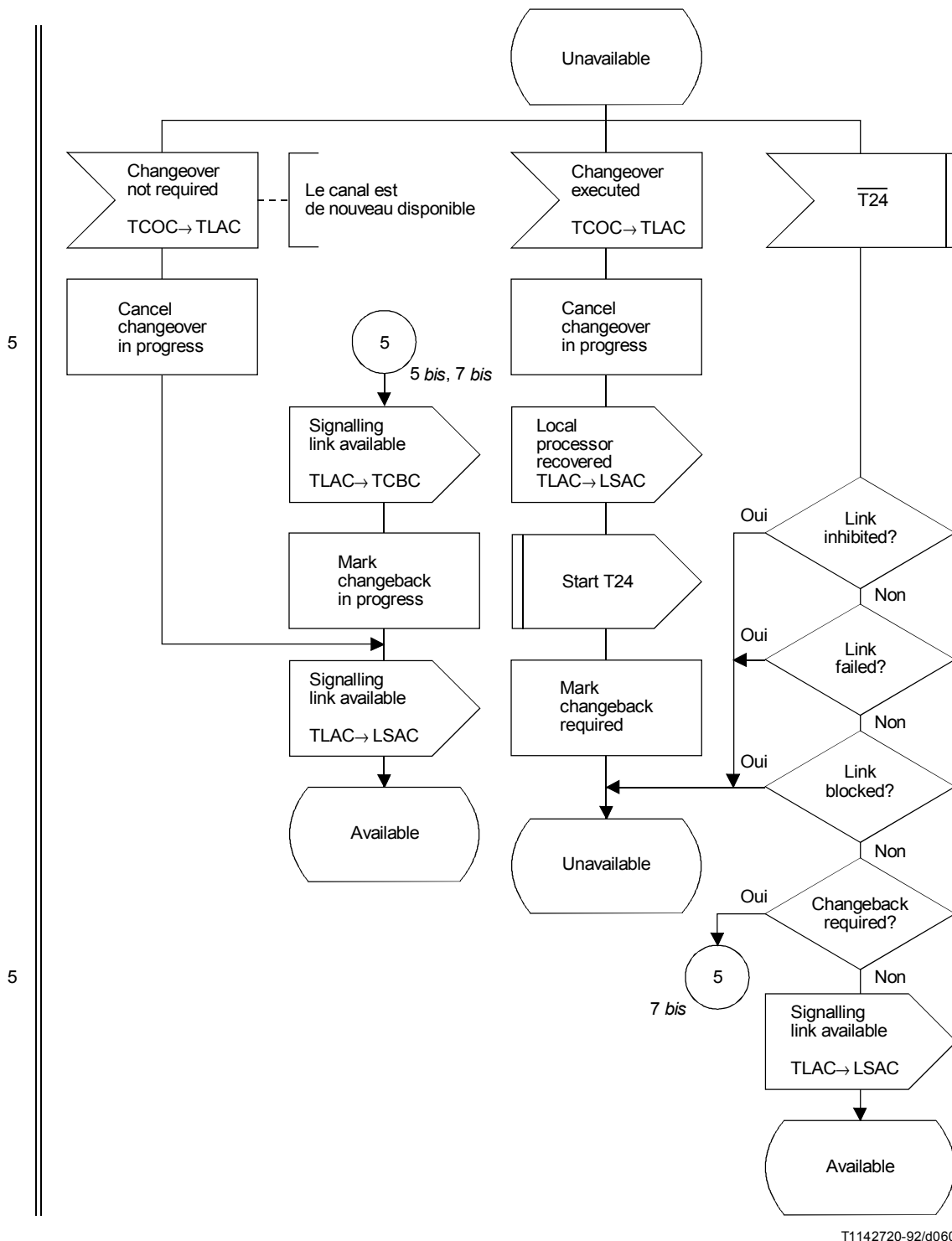
FIGURE 28/Q.704 (feuillet 7 bis sur 18) Gestion du trafic sémaphore; contrôle de la disponibilité des canaux sémaphores (TLAC) (option nationale)
