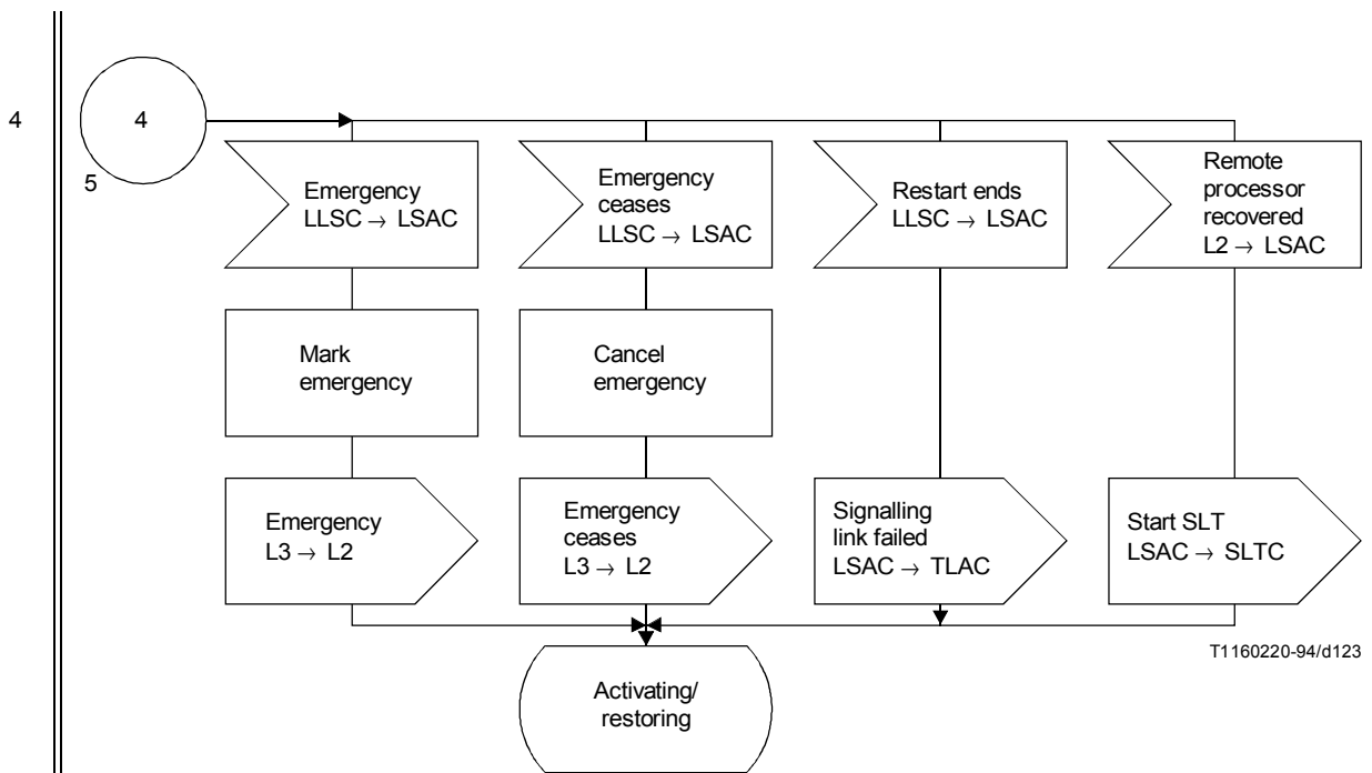
FIGURE 37/Q.704 (feuillet 6 sur 10) Gestion des canaux sémaphores; supervision de l'activité des canaux sémaphores (LSAC)
