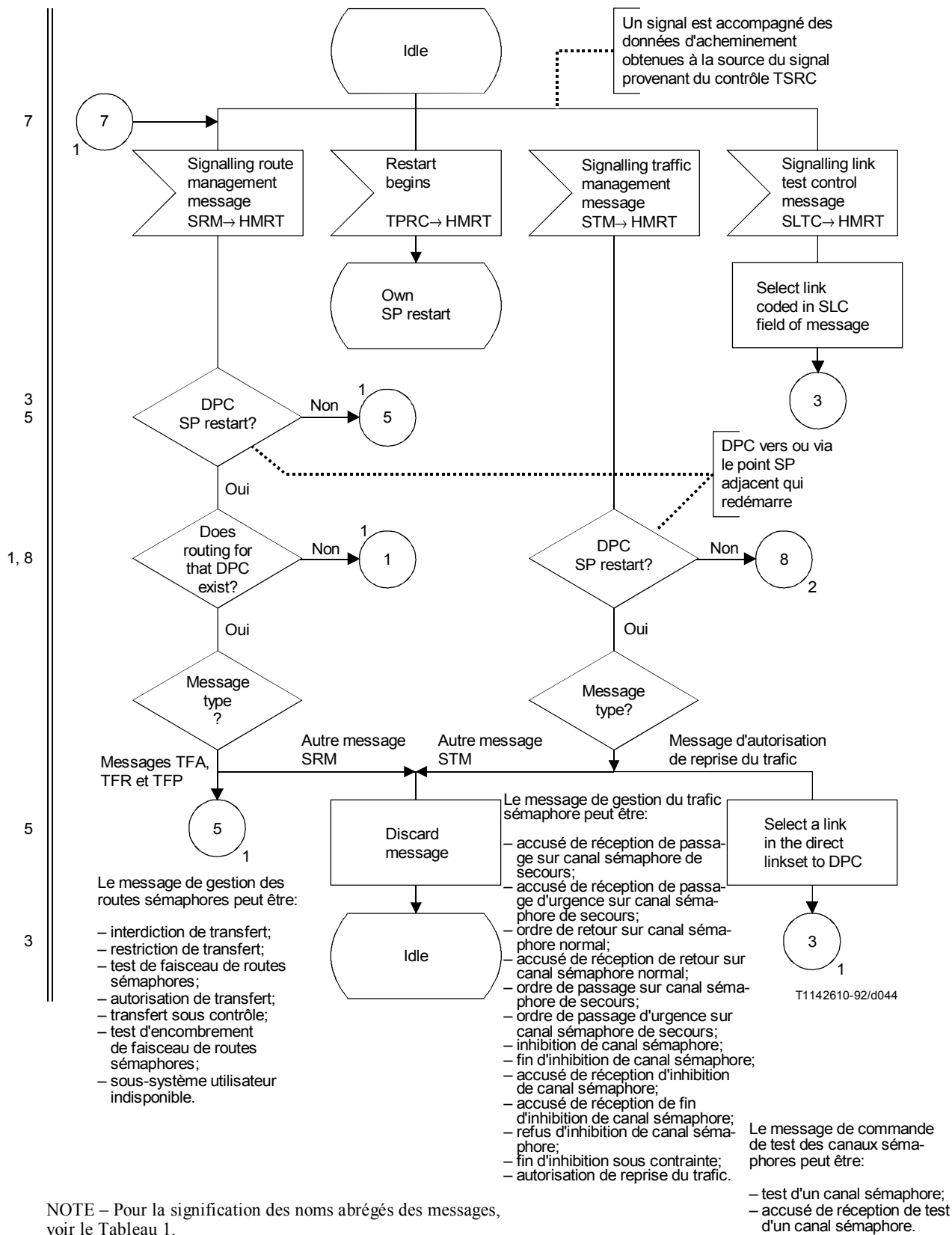
FIGURE 26/Q.704 (feuillet 3 sur 5)
