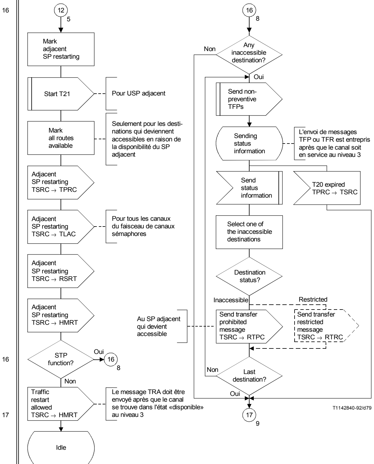
FIGURE 29/Q.704 (feuille 8 sur 21)
