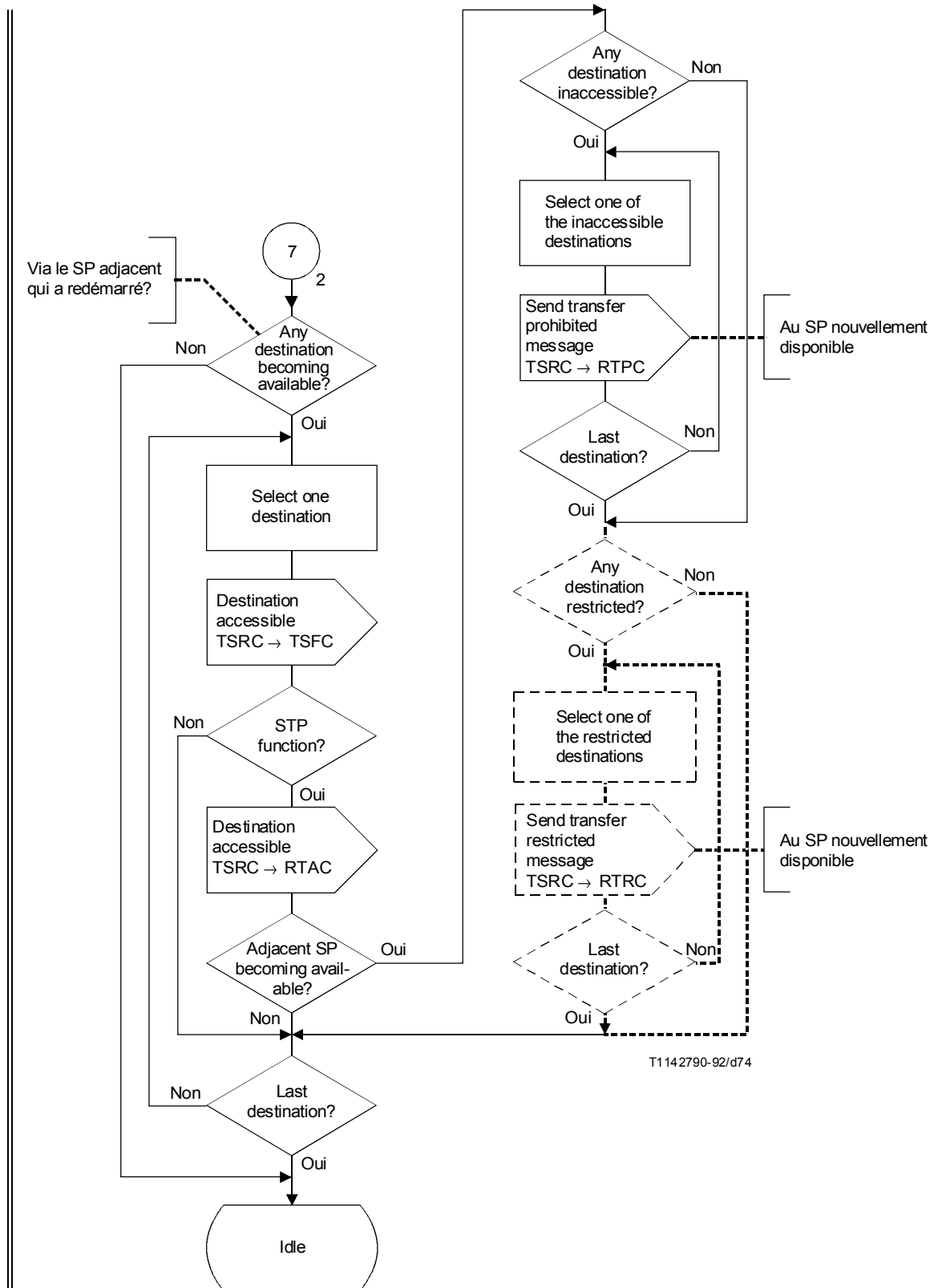
FIGURE 29/Q.704 (feuillet 3 sur 21)
