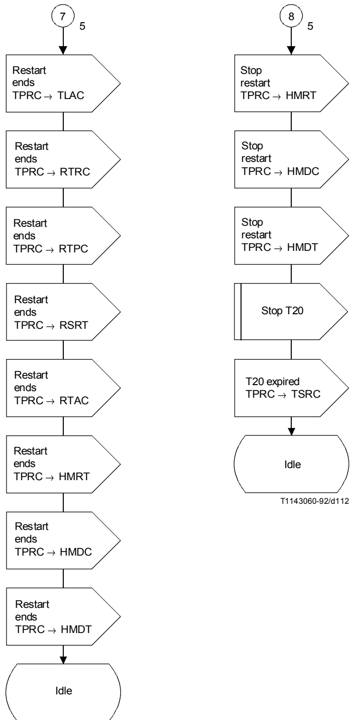
FIGURE 34b/Q.704 (feuillet 7 sur 7) Gestion du trafic sémaphore; commande de redémarrage d'un point sémaphore (TPRC)
