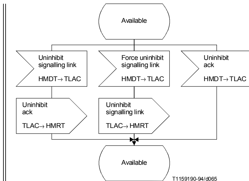
FIGURE 28/Q.704 (feuillet 12 sur 18) Gestion du trafic sémaphore; contrôle de la disponibilité des canaux sémaphores (TLAC)
