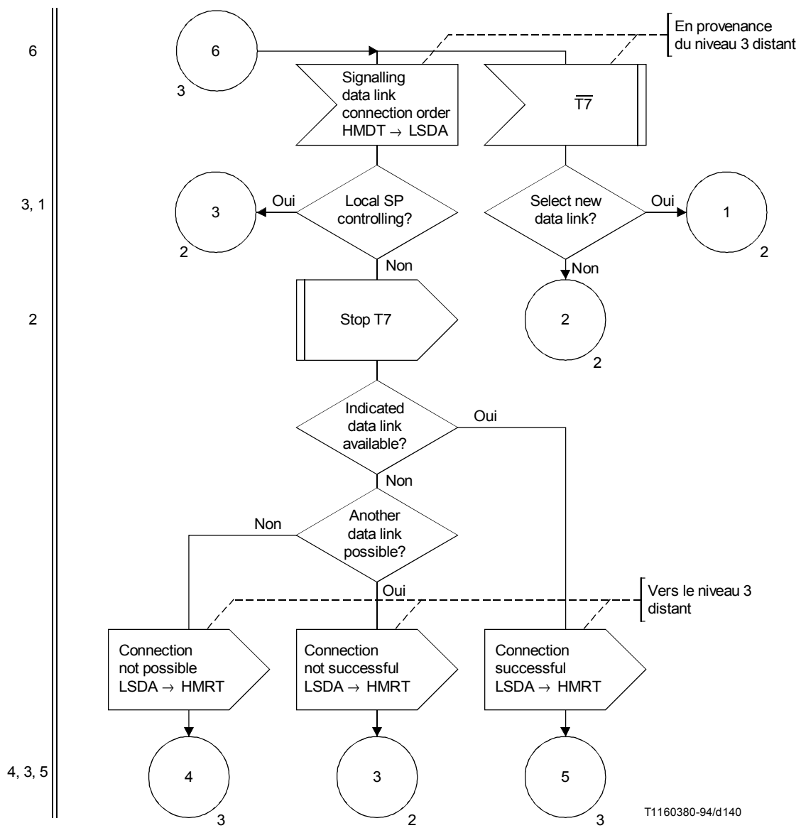
FIGURE 42/Q.704 (feuillet 4 sur 4)
