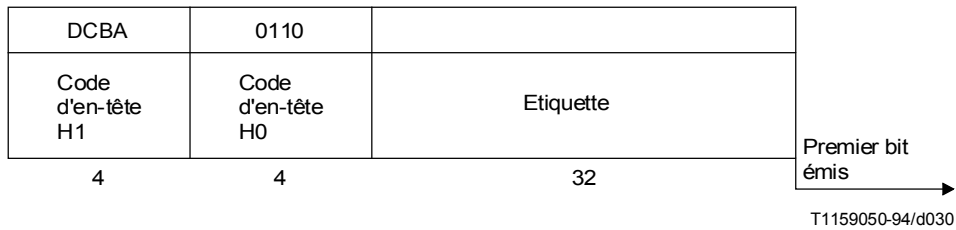
FIGURE 20a/Q.704 Message d'inhibition par la gestion
