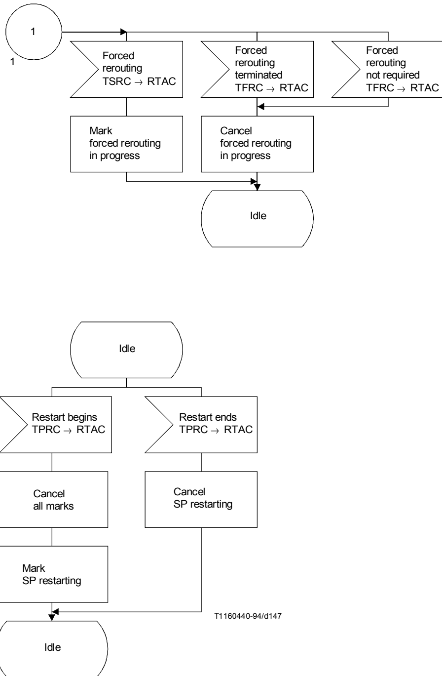
FIGURE 45/Q.704 (feuillet 2 sur 2)
