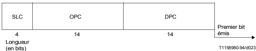
FIGURE 14/Q.704 Structure de l'étiquette normalisée
