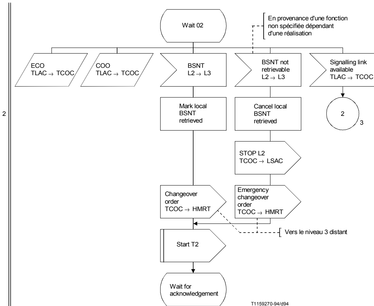
FIGURE 30/Q.704 (feuillet 2 sur 6) Gestion du trafic sémaphore; commande de passage sur canal sémaphore de secours (TCOC)
