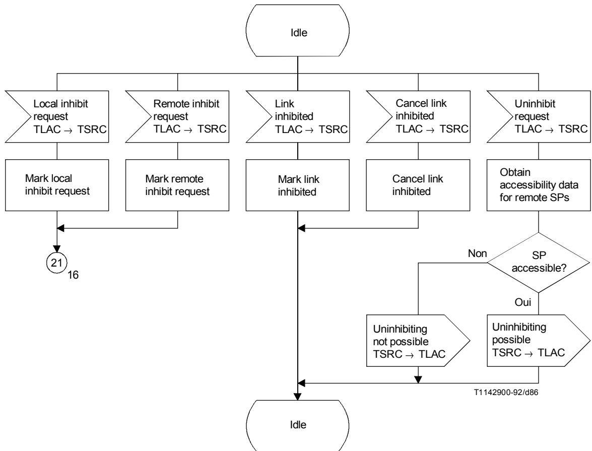
FIGURE 29/Q.704 (feuillet 15 sur 21) Gestion du trafic sémaphore; commande des acheminements de la signalisation (TSRC)
