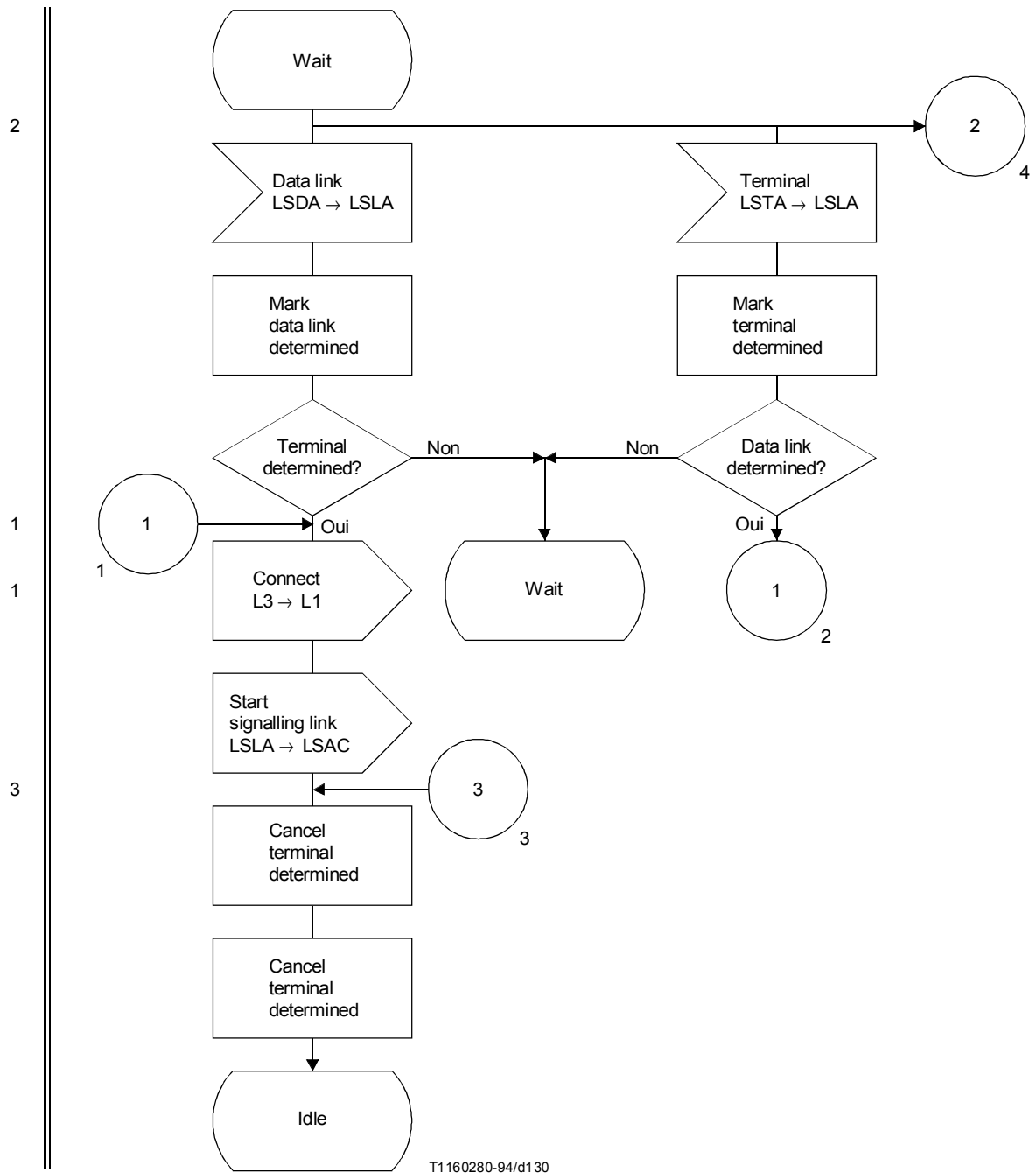
FIGURE 38/Q.704 (feuillet 2 sur 3)
