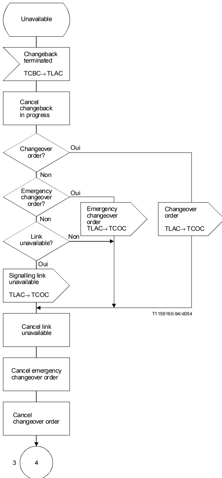
FIGURE 28/Q.704 (feuillet 4 sur 18)
