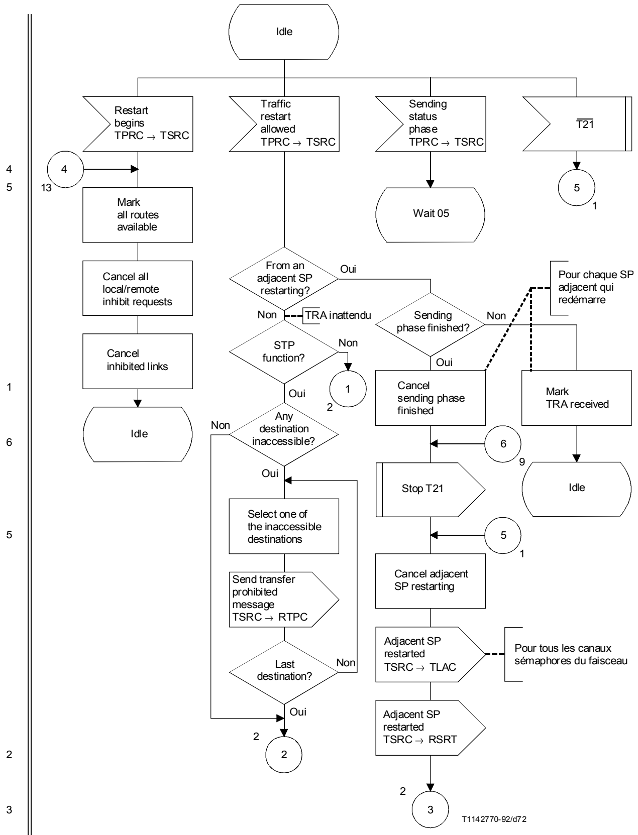
FIGURE 29/Q.704 (feuillet 1 sur 21)
