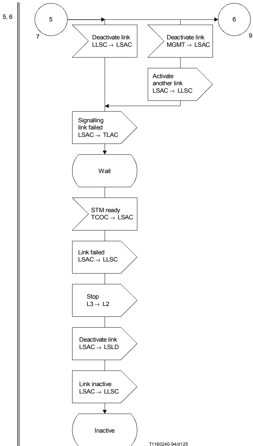
FIGURE 37/Q.704 (feuillet 8 sur 10)
