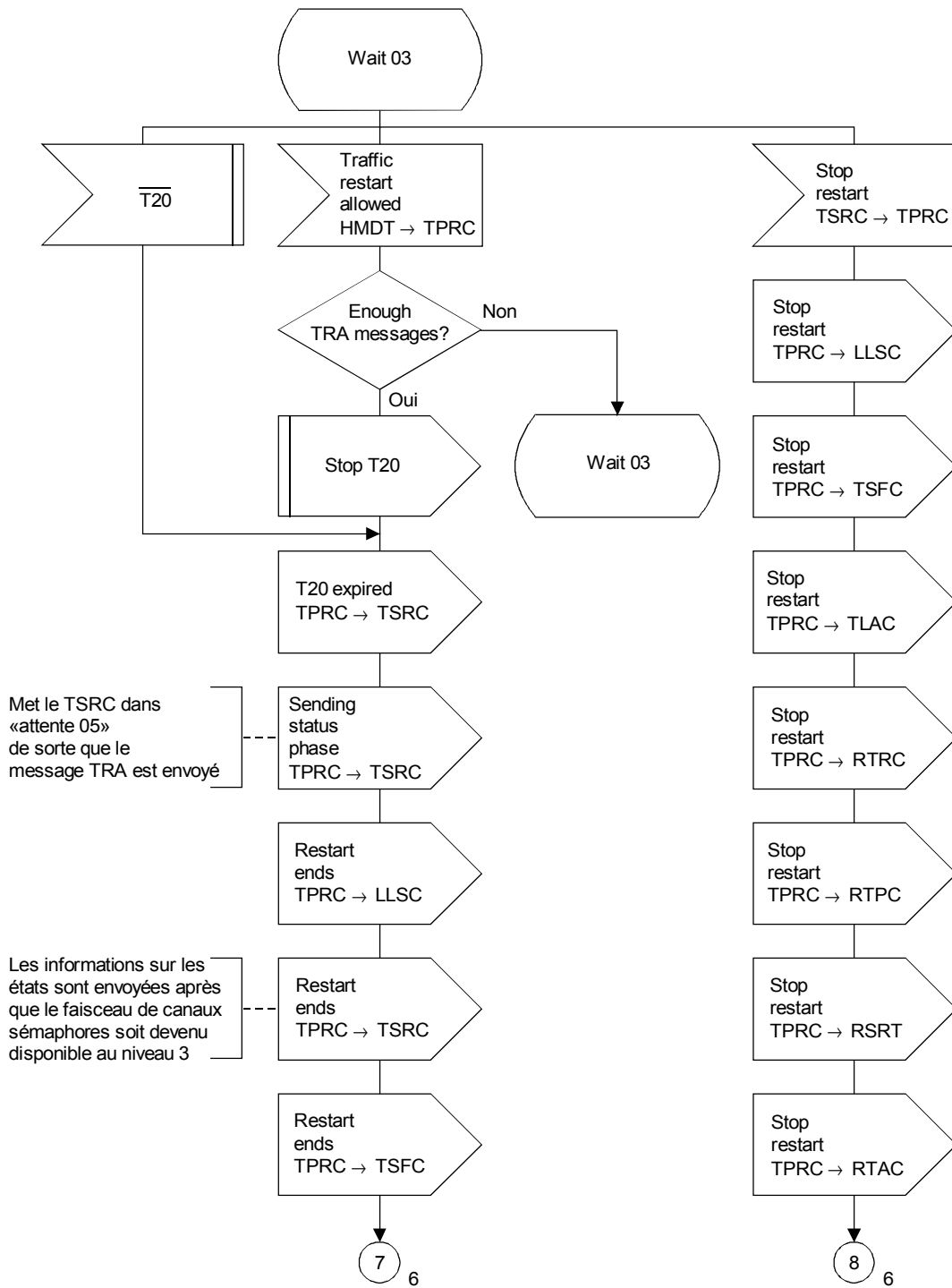
FIGURE 34b/Q.704 (feuillet 6 sur 7)
