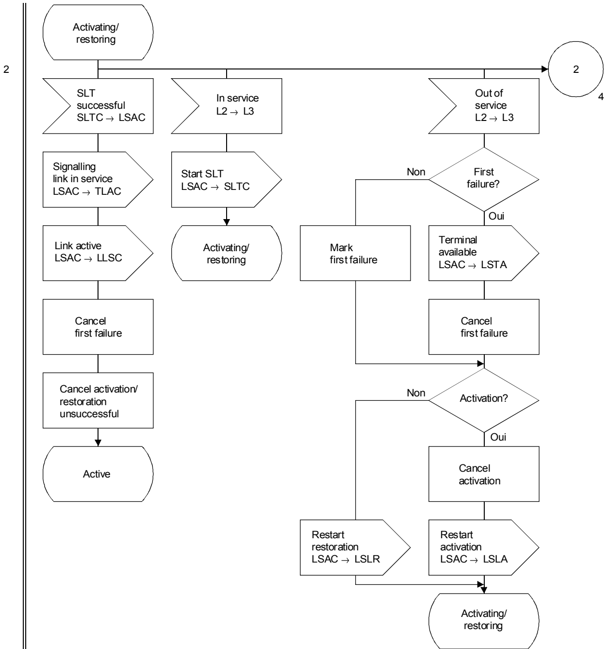
FIGURE 37/Q.704 (feuillet 3 sur 10)
