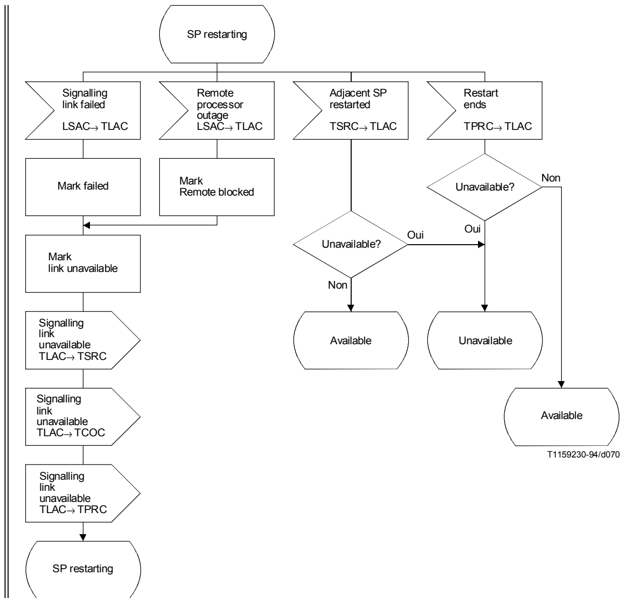
FIGURE 28/Q.704 (feuille 17 sur 18) Gestion du trafic sémaphore; contrôle de la disponibilité des canaux sémaphores (TLAC)
