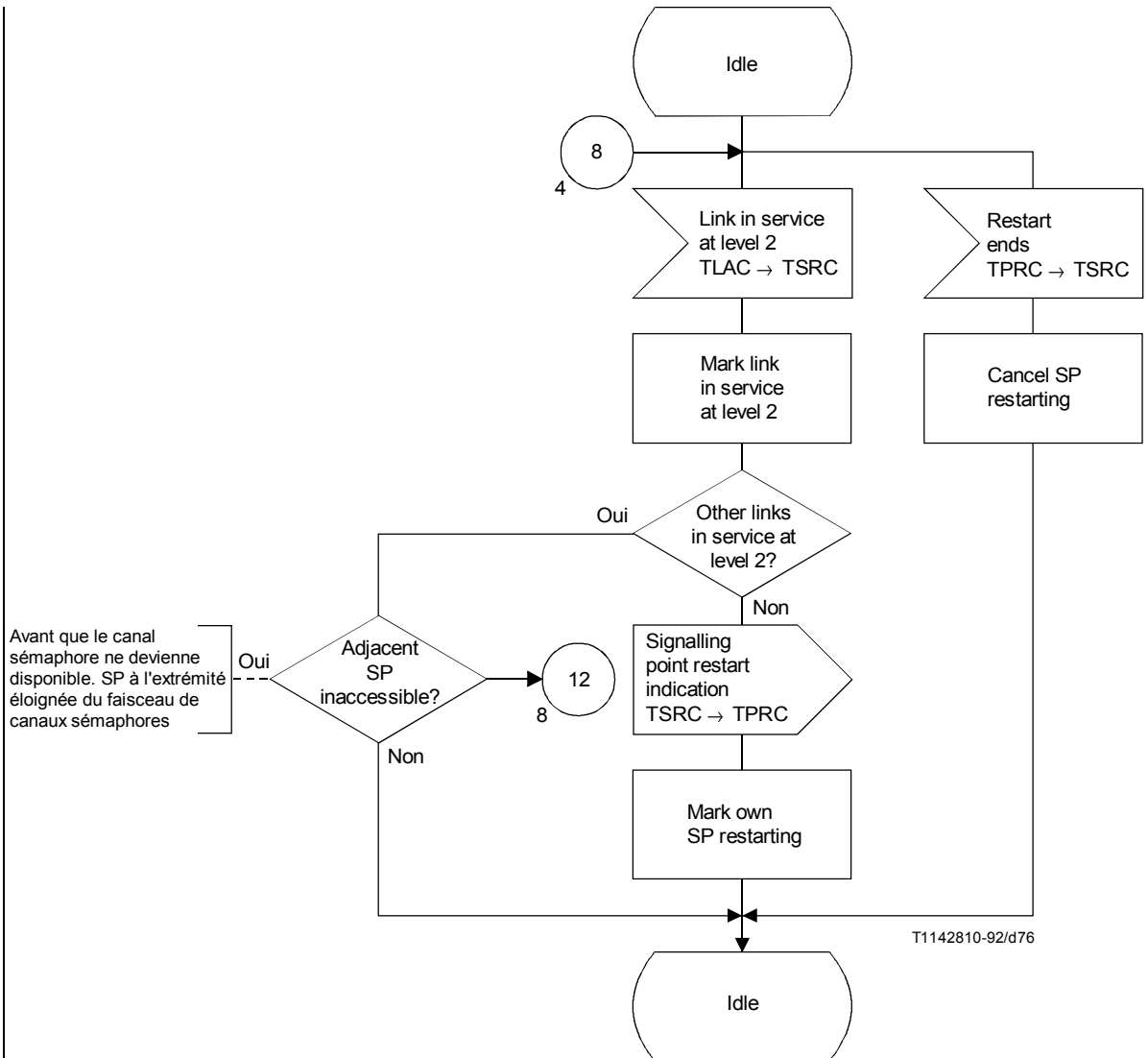
FIGURE 29/Q.704 (feuillet 5 sur 21)
