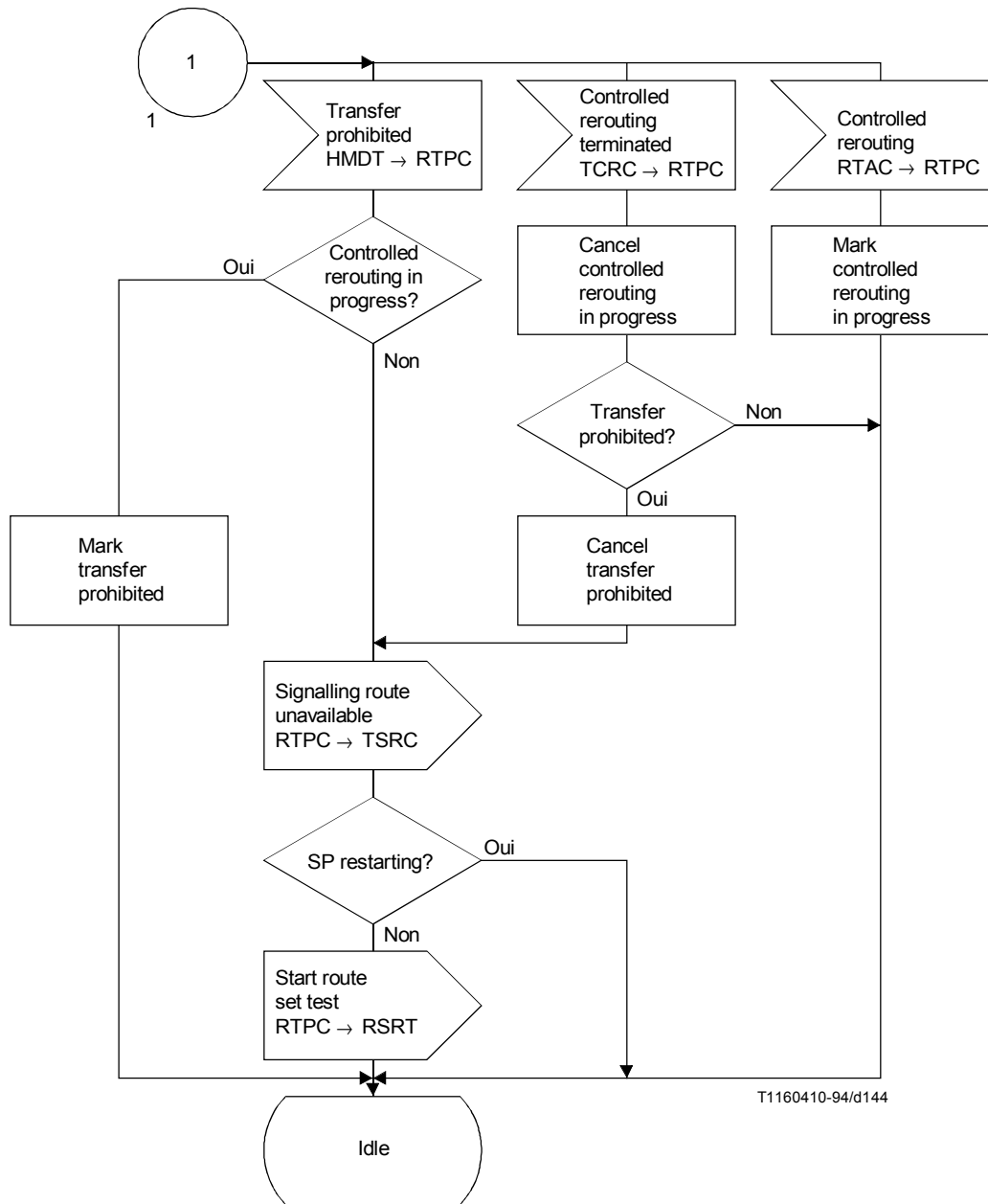
FIGURE 44/Q.704 (feuillet 2 sur 3) Gestion des routes sémaphores; commande d'interdiction de transfert (RTPC)
