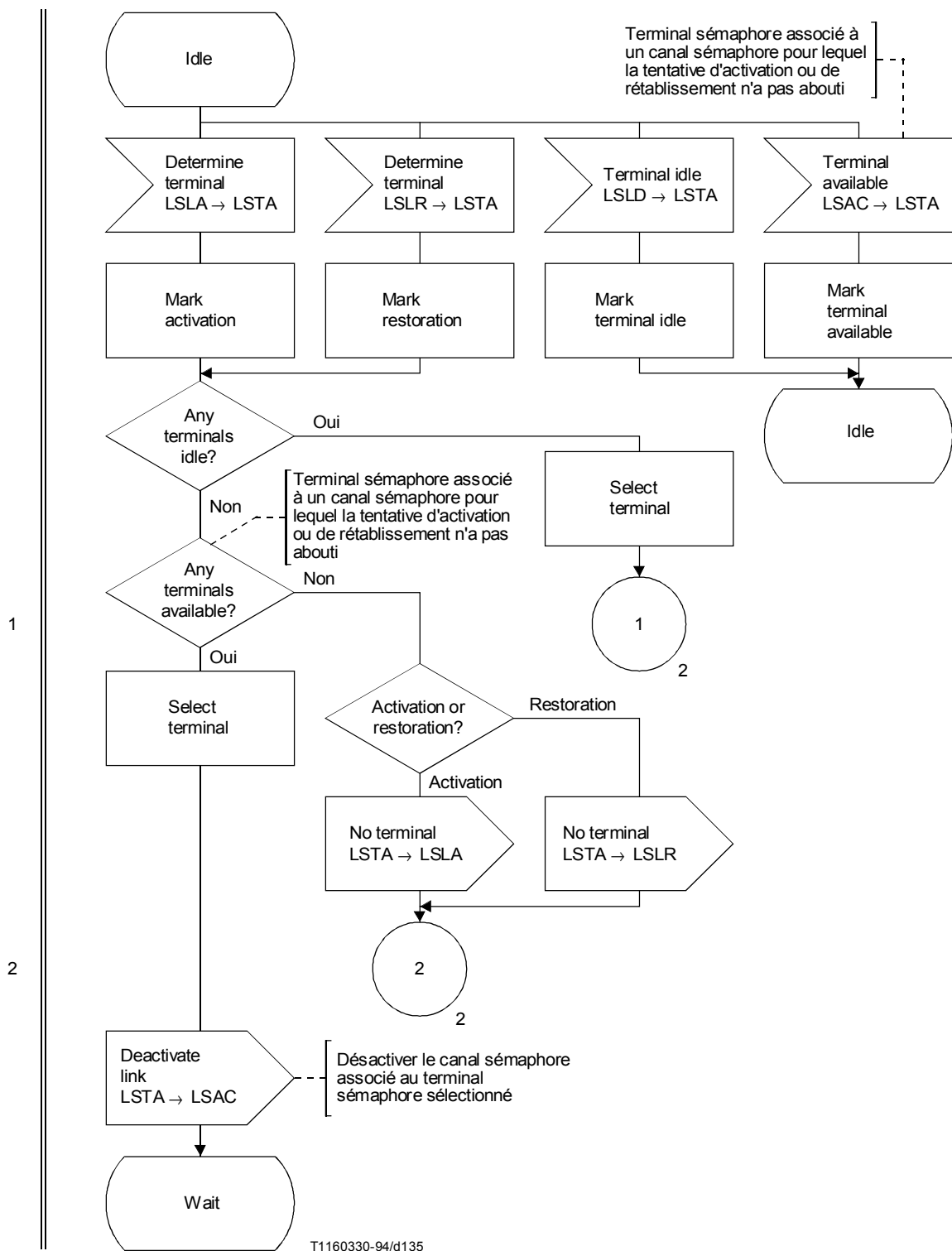
FIGURE 41/Q.704 (feuillet 1 sur 2)
