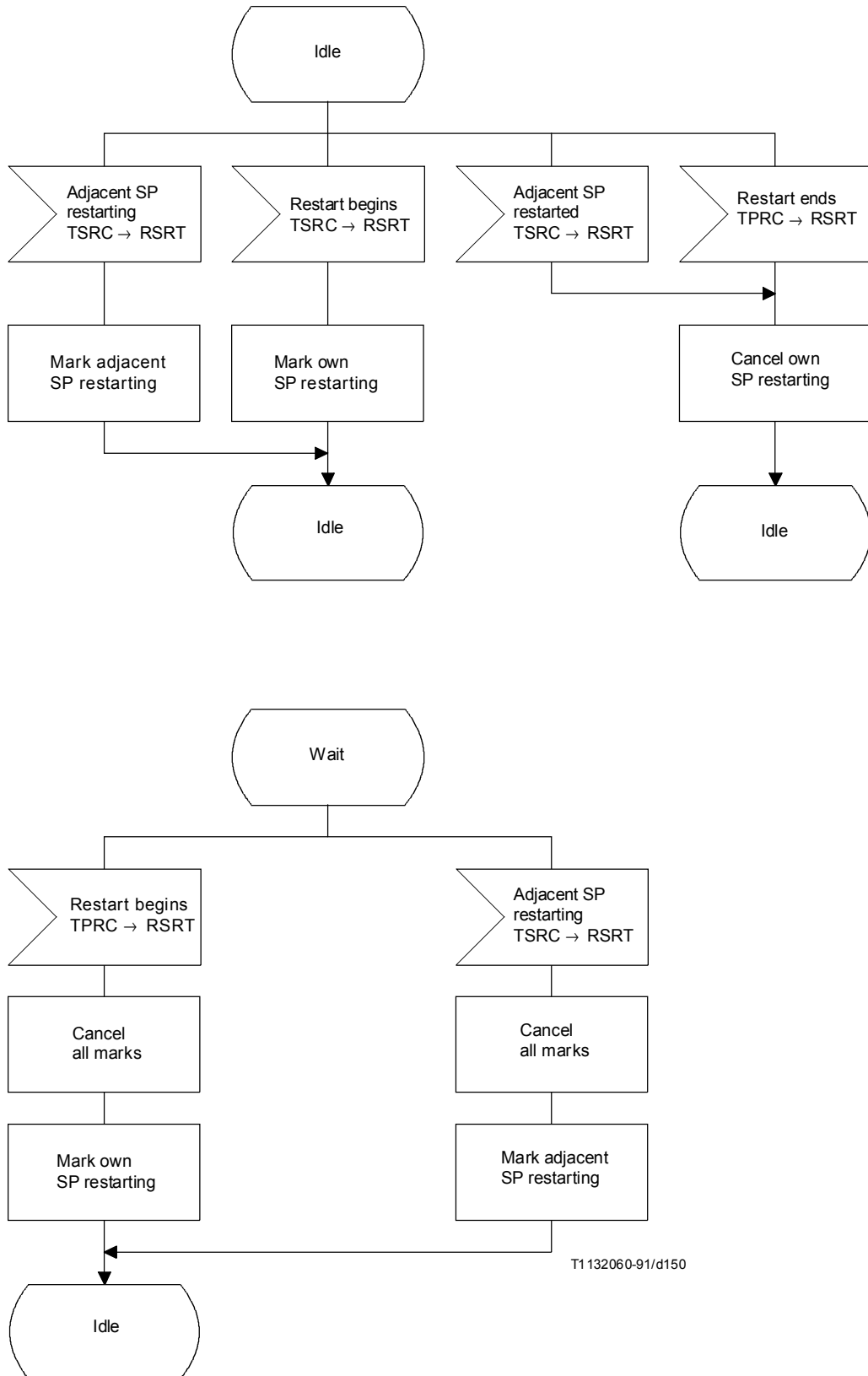
FIGURE 46/Q.704 (feuillet 3 sur 3)
