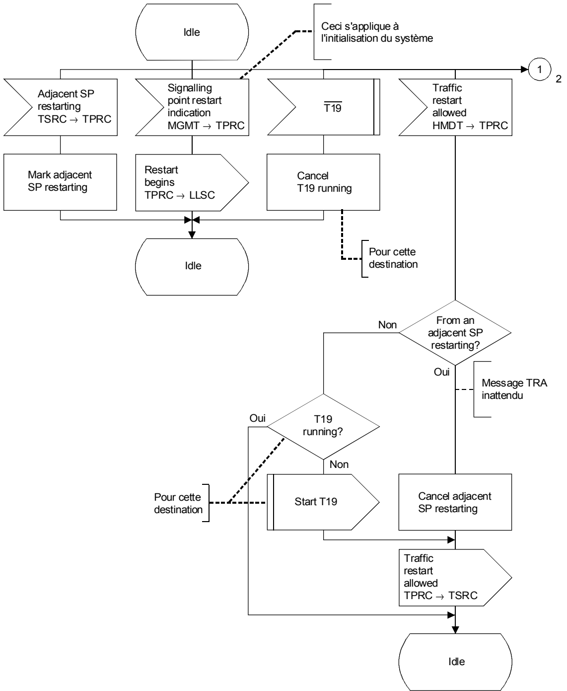
FIGURE 34b/Q.704 (feuillet 1 sur 7) Gestion du trafic sémaphore; commande de redémarrage d'un point sémaphore (TPRC)
