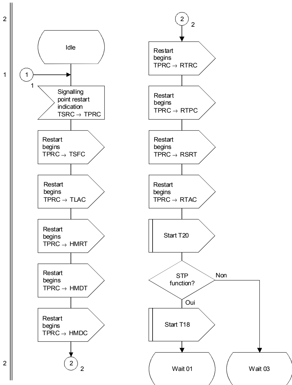
FIGURE 34b/Q.704 (feuillet 2 sur 7)
