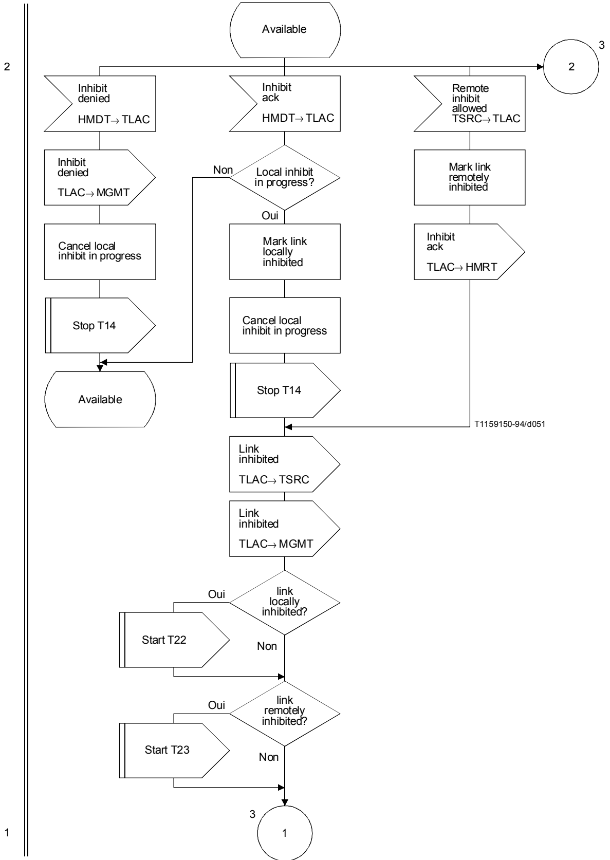
FIGURE 28/Q.704 (feuillet 2 sur 18)
