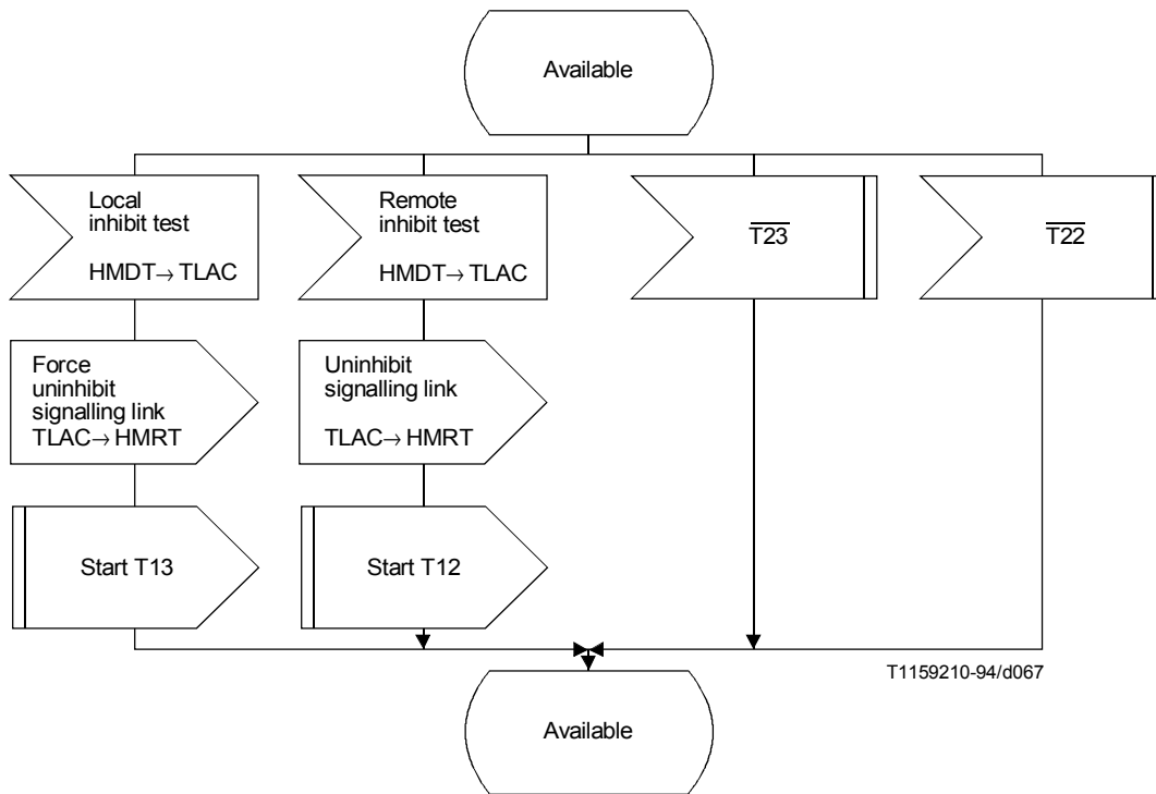
FIGURE 28/Q.704 (feuille 14 sur 18) Gestion du trafic sémaphore; contrôle de la disponibilité des canaux sémaphores (TLAC)
