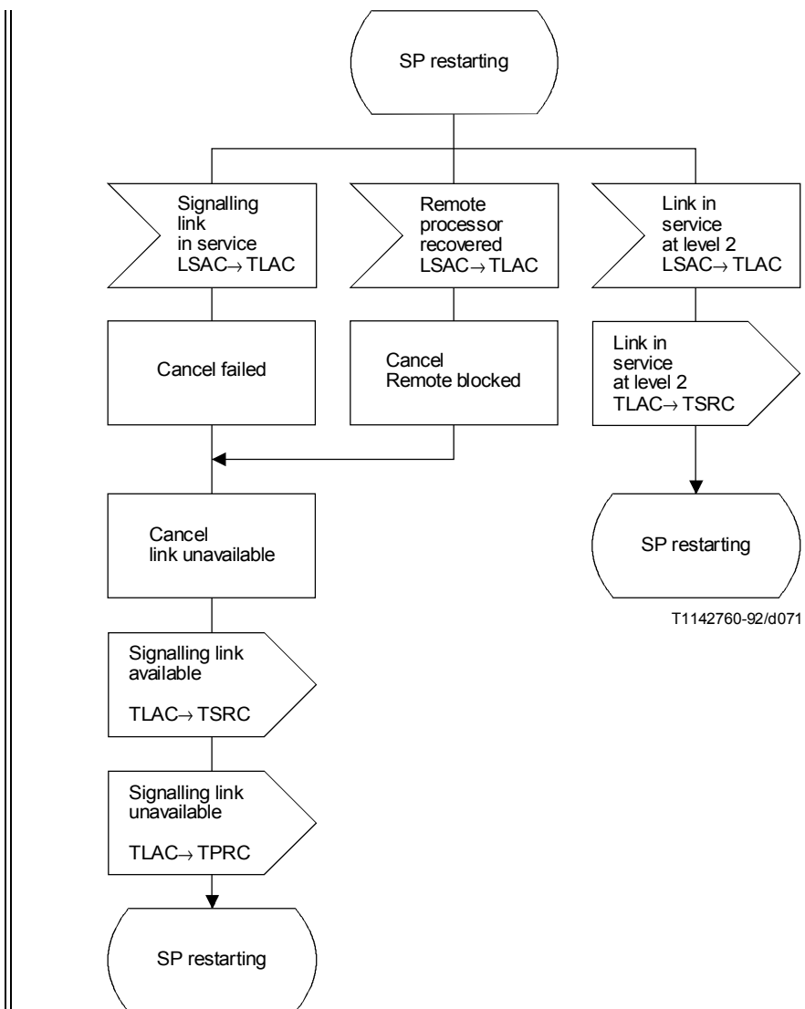
FIGURE 28/Q.704 (feuille 18 sur 18) Gestion du trafic sémaphore; contrôle de la disponibilité des canaux sémaphores (TLAC)
