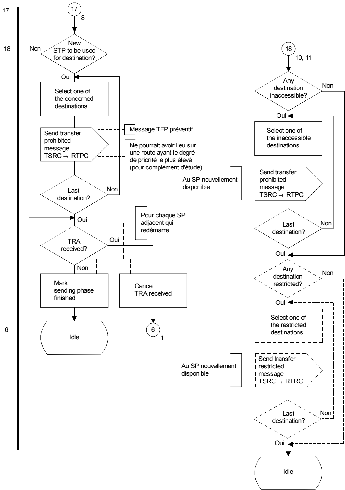
FIGURE 29/Q.704 (feuillet 9 sur 21)
