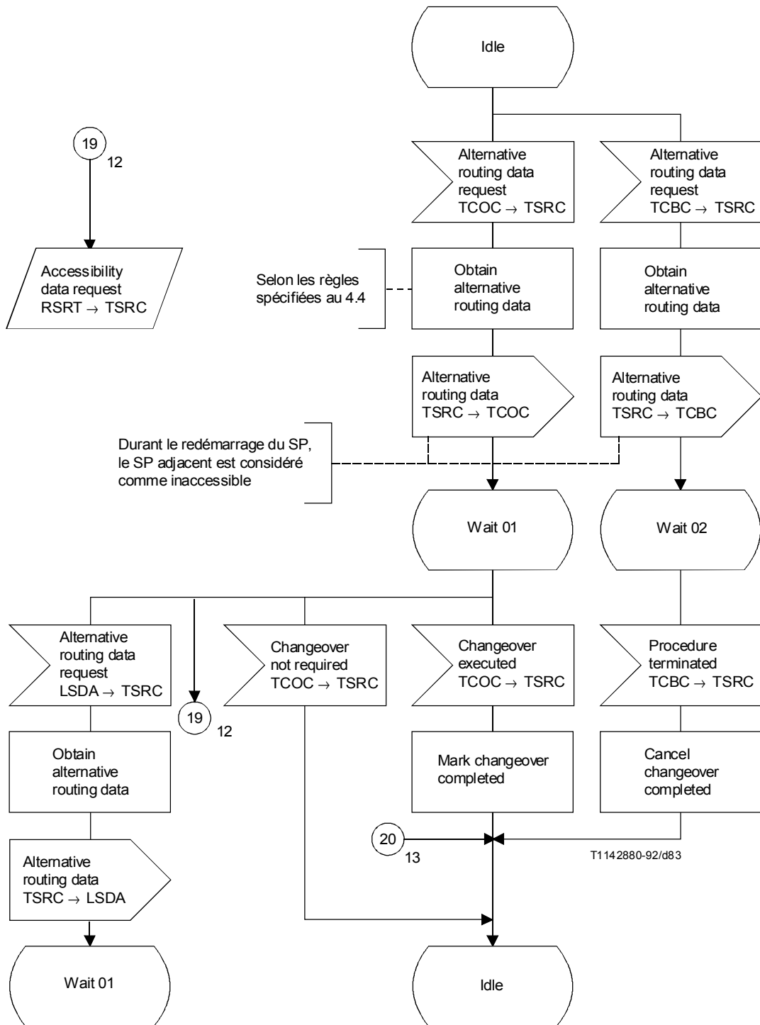
FIGURE 29/Q.704 (feuille 12 sur 21)
