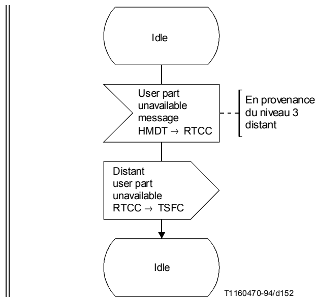
FIGURE 46a/Q.704 (feuillet 2 sur 2) Gestion des routes sémaphores; commande de transfert sous contrôle (RTCC)
