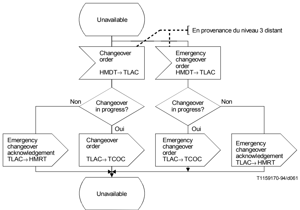
FIGURE 28/Q.704 (feuillet 8 sur 18)
