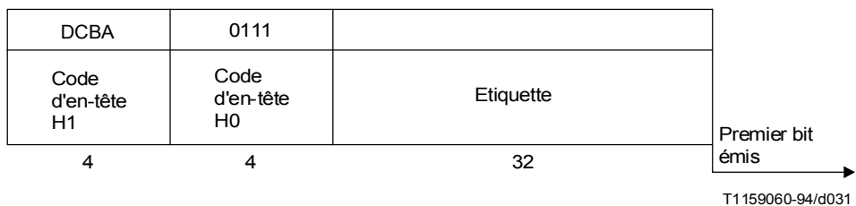
FIGURE 21/Q.704 Message d'autorisation de reprise du trafic
