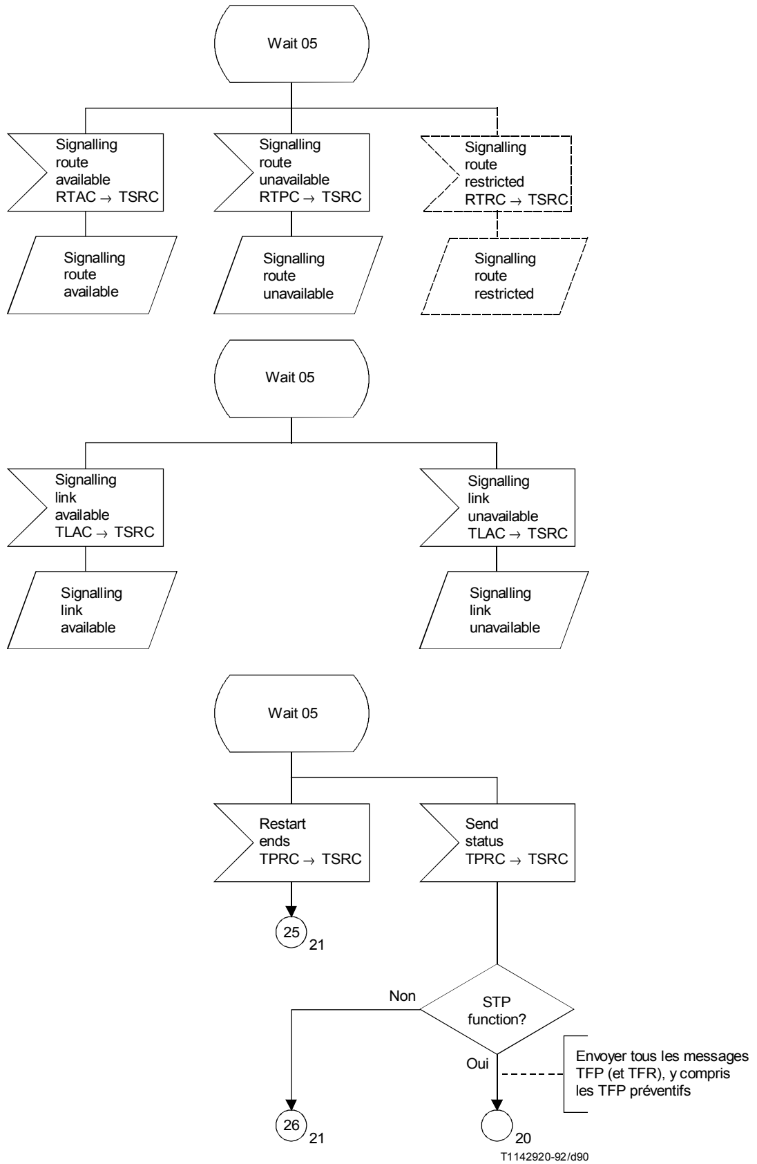
FIGURE 29/Q.704 (feuillet 19 sur 21)
