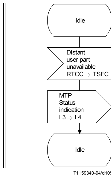
FIGURE 34a/Q.704 (feuillet 3 sur 3) Gestion du trafic sémaphore; contrôle de flux de trafic sémaphore (TSFC)
