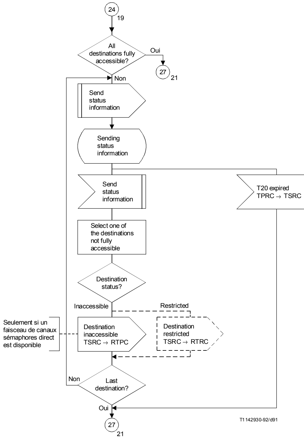
FIGURE 29/Q.704 (feuillet 20 sur 21) Gestion du trafic sémaphore; contrôle des acheminements de la signalisation (TSRC)
