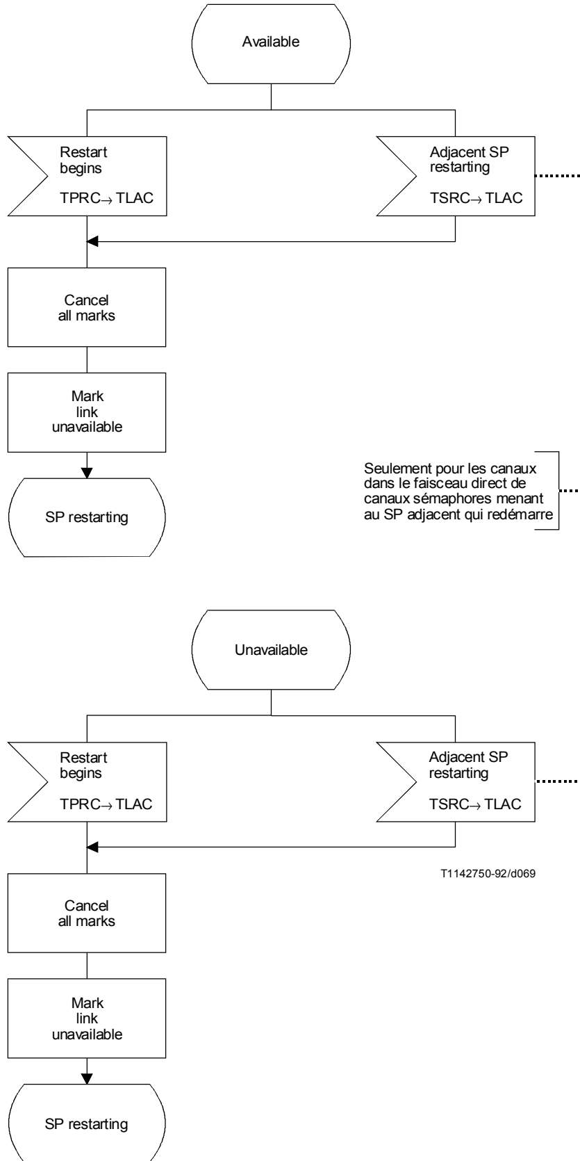
FIGURE 28/Q.704 (feuille 16 sur 18) Gestion du trafic sémaphore; contrôle de la disponibilité des canaux sémaphores (TLAC)
