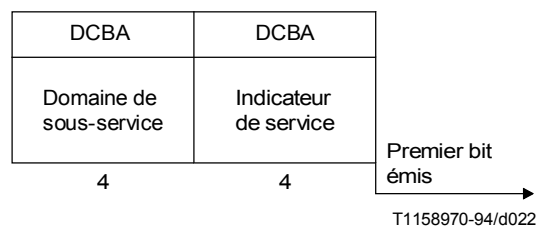
FIGURE 13/Q.704 Octet d'information de service
