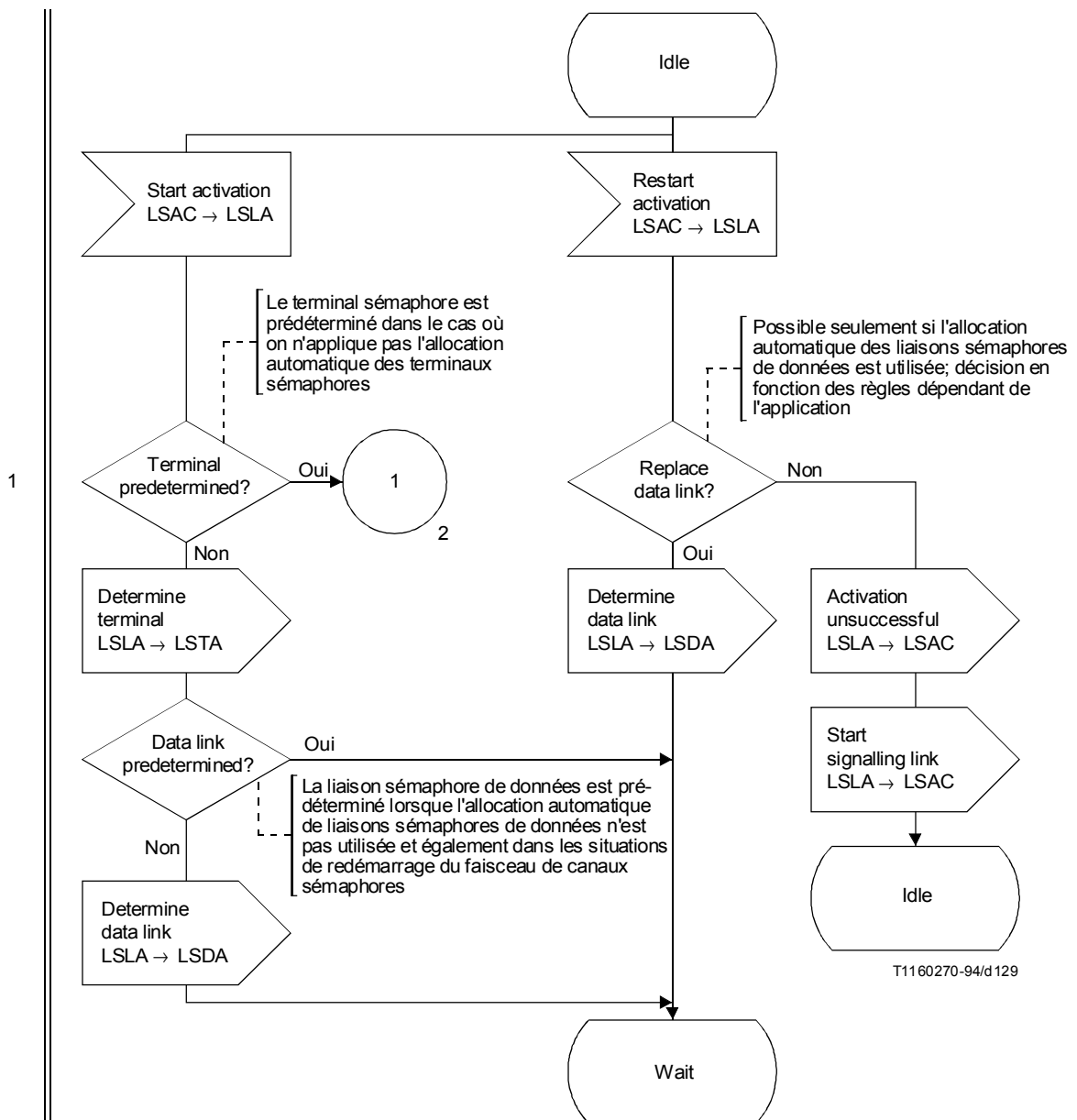
FIGURE 38/Q.704 (feuillet 1 sur 3)
