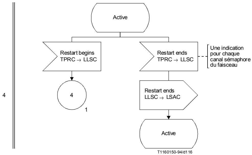
FIGURE 36/Q.704 (feuillet 3 sur 3) Gestion des canaux sémaphores; contrôle des faisceaux de canaux sémaphores (LLSC)
