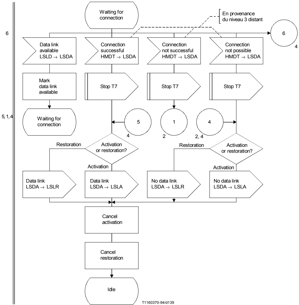
FIGURE 42/Q.704 (feuillet 3 sur 4)
