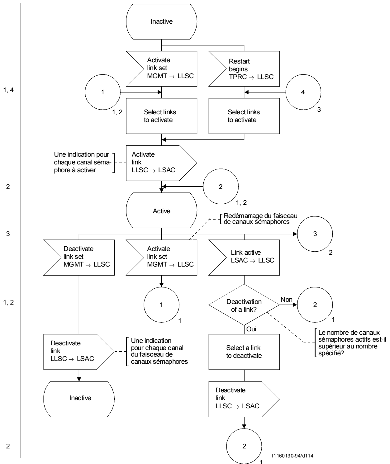
FIGURE 36/Q.704 (feuille 1 sur 3)
