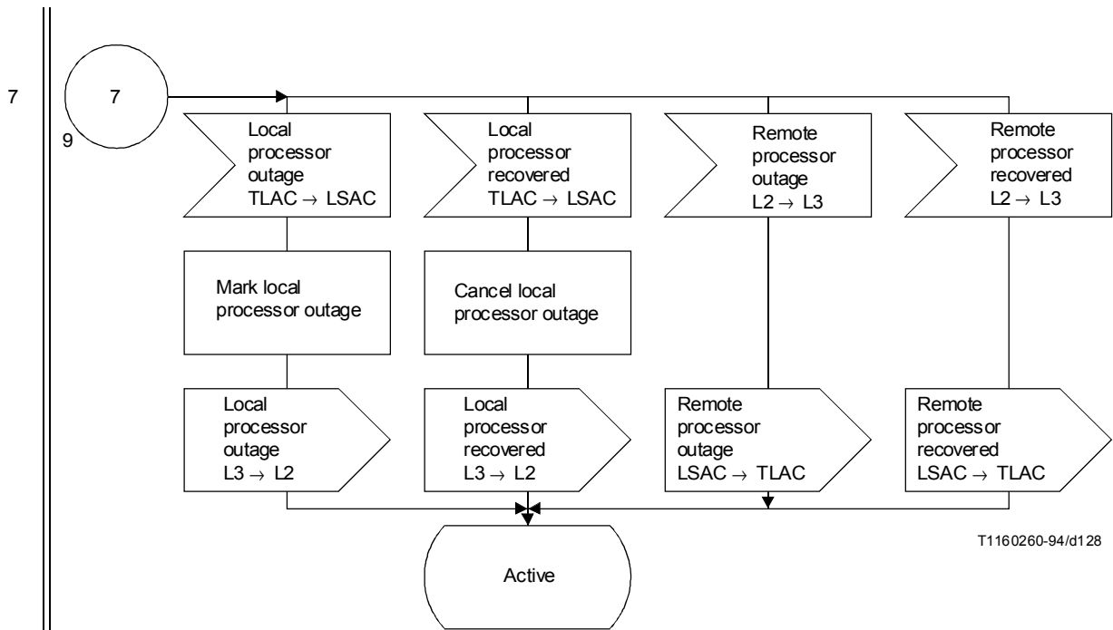
FIGURE 37/Q.704 (feuillet 10 bis sur 10)
