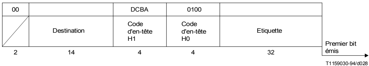
FIGURE 19/Q.704 Message d'autorisation de transfert
