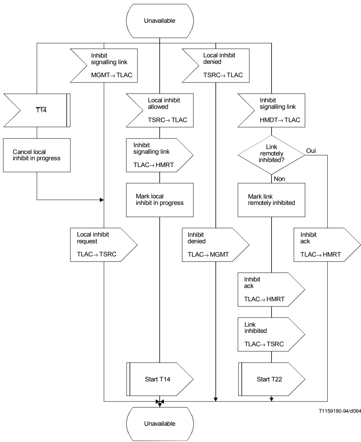
FIGURE 28/Q.704 (feuillet 11 sur 18) Gestion du trafic sémaphore; contrôle de la disponibilité des canaux sémaphores (TLAC)
