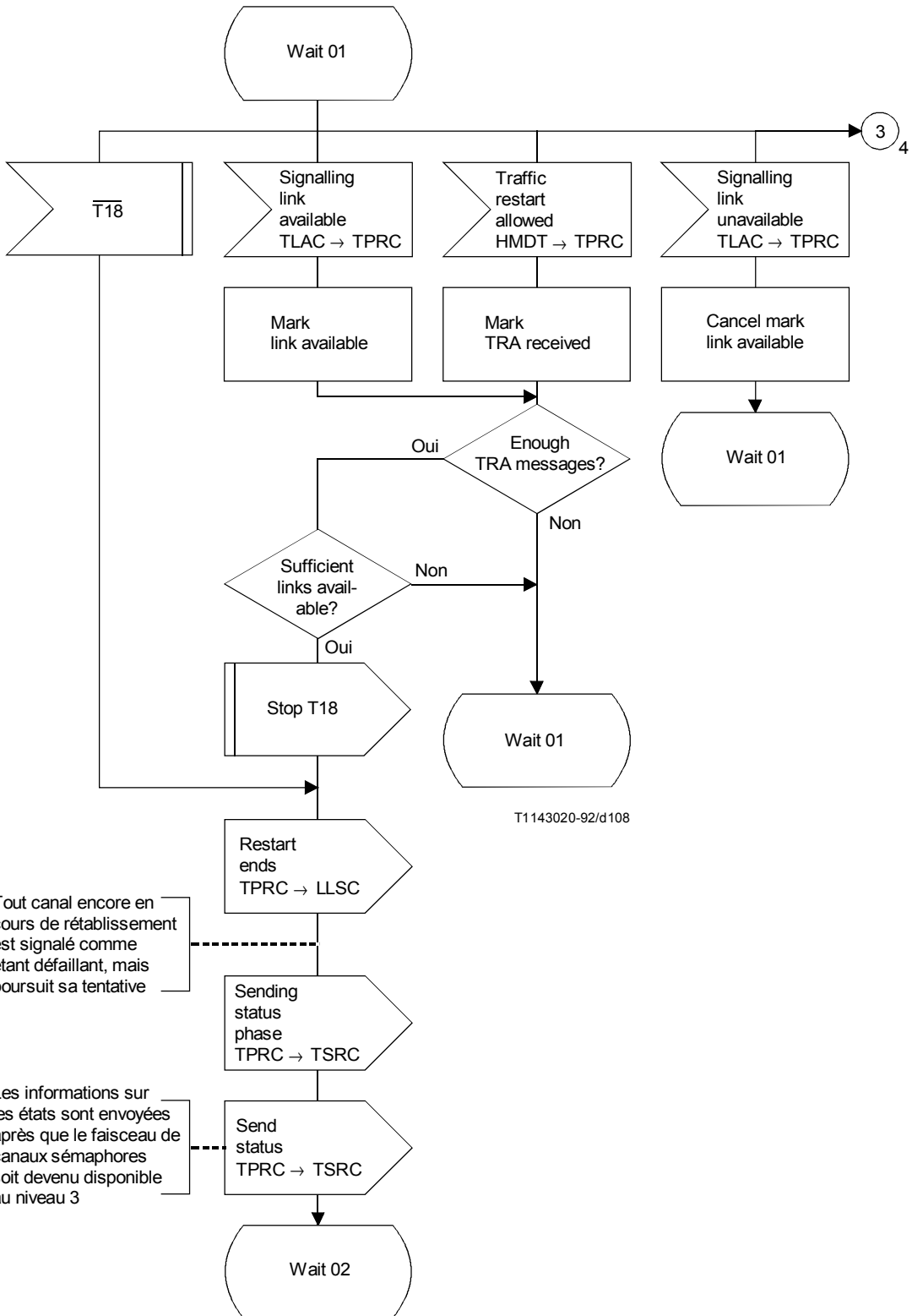
FIGURE 34b/Q.704 (feuillet 3 sur 7) Gestion du trafic sémaphore; commande de redémarrage d'un point sémaphore (TPRC)
