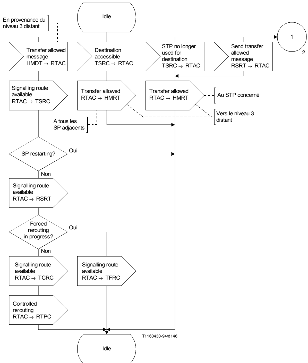
FIGURE 45/Q.704 (feuillet 1 sur 2)
