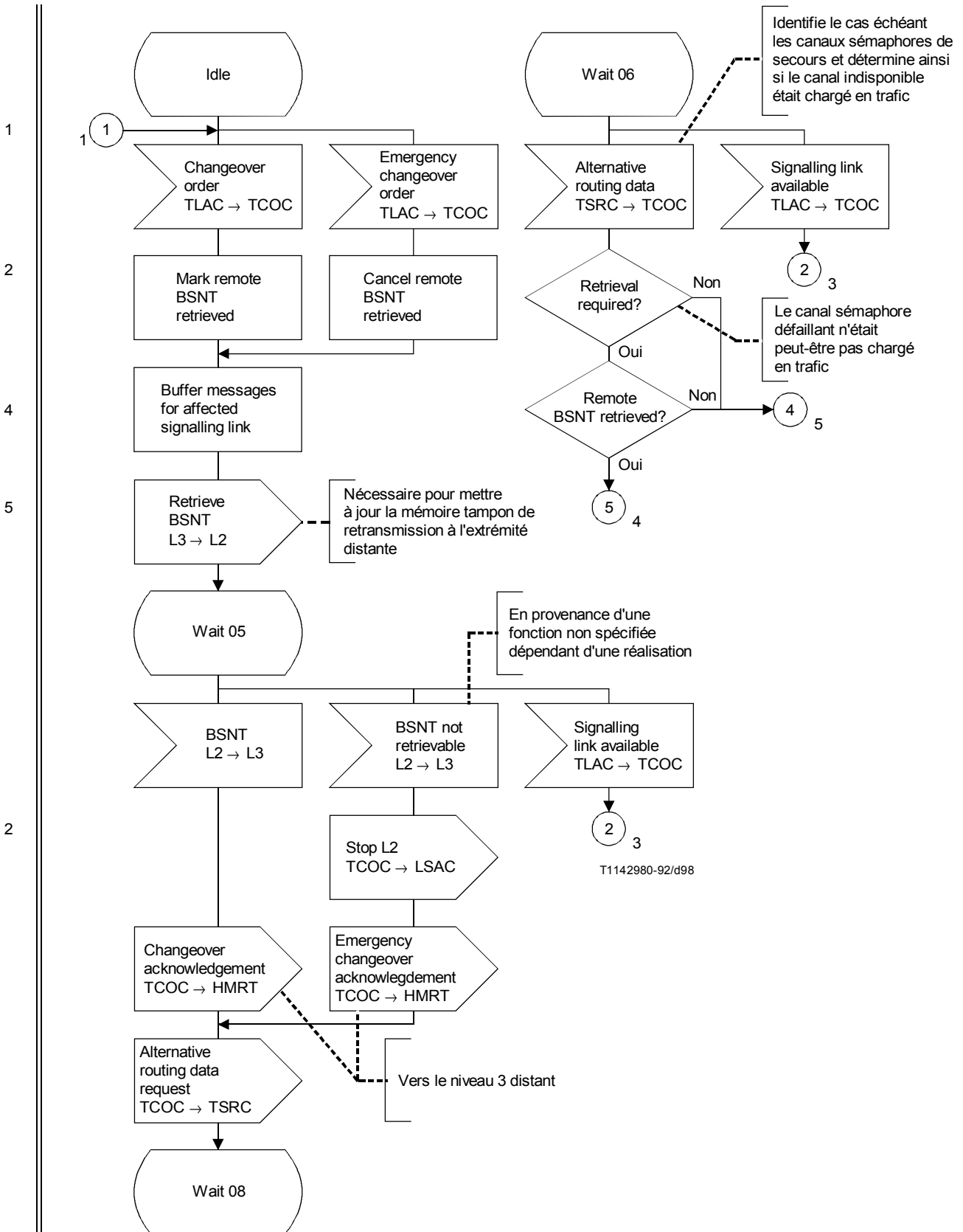
FIGURE 30/Q.704 (feuillet 6 sur 6)
