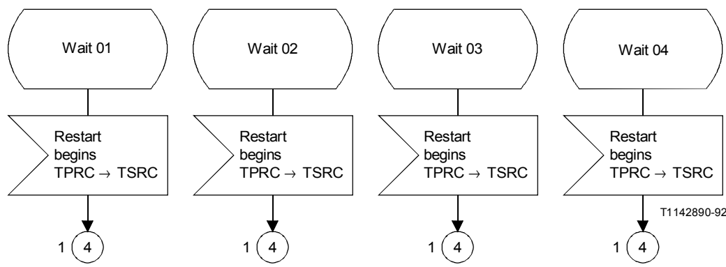
FIGURE 29/Q.704 (feuillet 13 sur 21)
