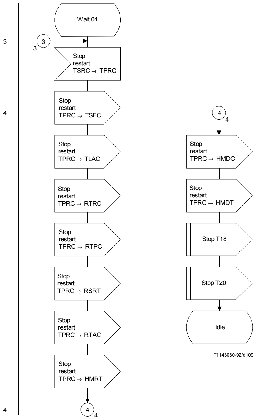
FIGURE 34b/Q.704 (feuillet 4 sur 7) Gestion du trafic sémaphore; commande de redémarrage d'un point sémaphore (TPRC)
