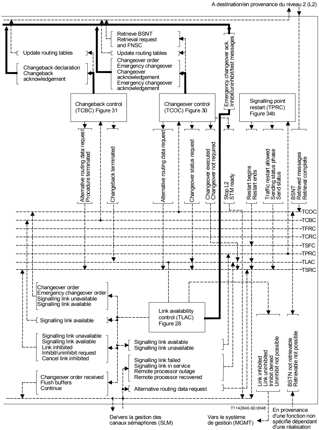
FIGURE 27/Q.704 (feuille 2 sur 3)
