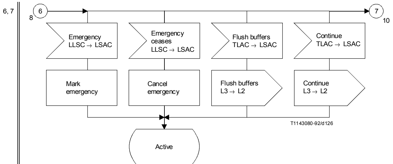
FIGURE 37/Q.704 (feuillet 9 sur 10)
