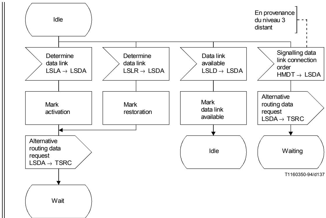
FIGURE 42/Q.704 (feuille 1 sur 4)
