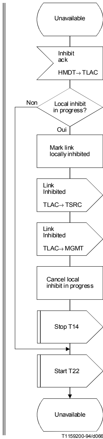
FIGURE 28/Q.704 (feuillet 13 sur 18) Gestion du trafic sémaphore; contrôle de la disponibilité des canaux sémaphores (TLAC)
