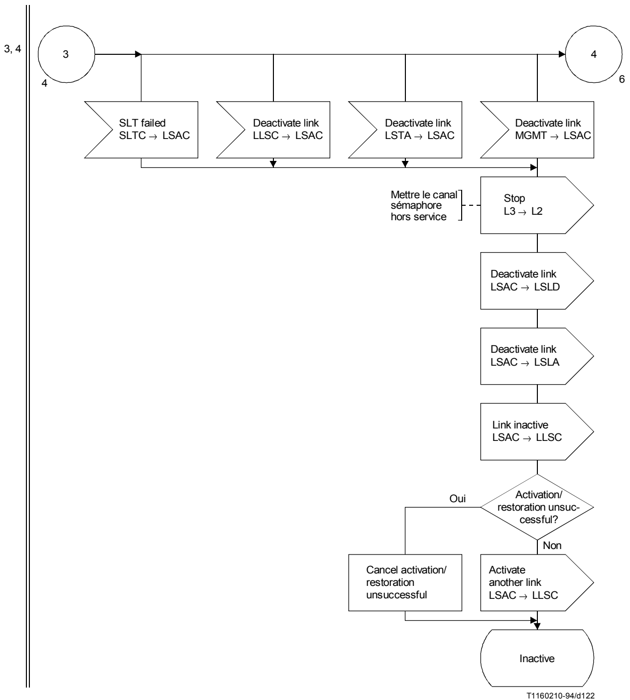
FIGURE 37/Q.704 (feuille 5 sur 10)
