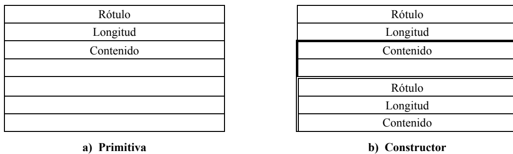
Figura B.4/Q.763 – Tipos de contenido
