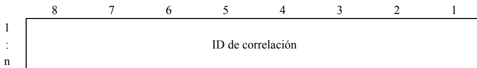
Figura 67/Q.763 – Campo del parámetro ID de correlación
