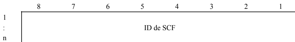
Figura 68/Q.763 – Campo del parámetro ID de SCF
