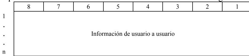
Figura 58/Q.763 – Campo del parámetro información de usuario a usuario
