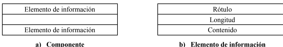
Figura B.1/Q.763 – Estructura de componente y elemento de información
