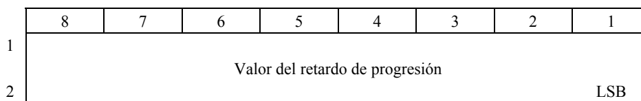
Figura 42/Q.763 – Campo del parámetro contador de retardo de propagación
