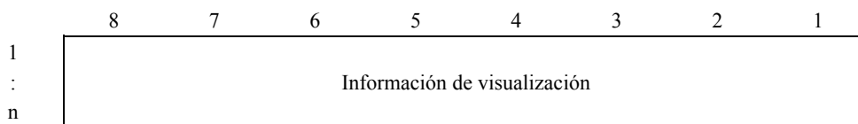
Figura 72/Q.763 – Campo del parámetro información de visualización
