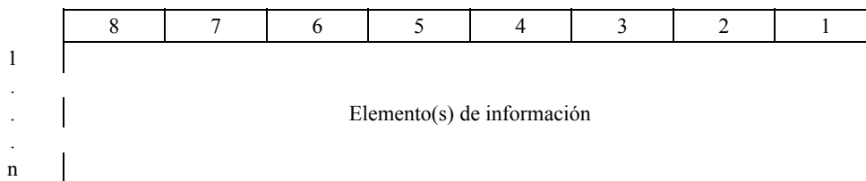
Figura 5/Q.763 – Campo del parámetro transporte de acceso
