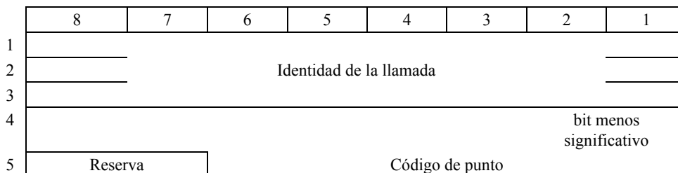
Figura 9/Q.763 – Campo del parámetro referencia de llamada
