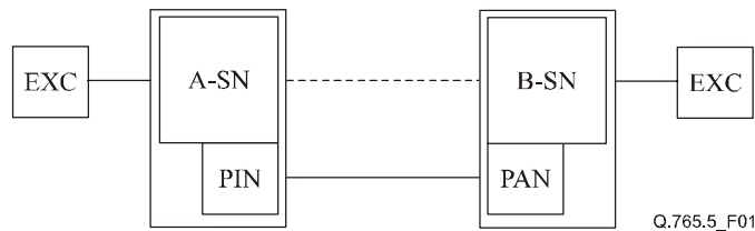
Figure 1/Q.765.5 – Topologie de réseau BICC
