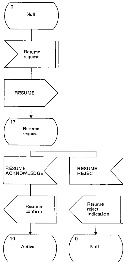
f) Resume procedure
