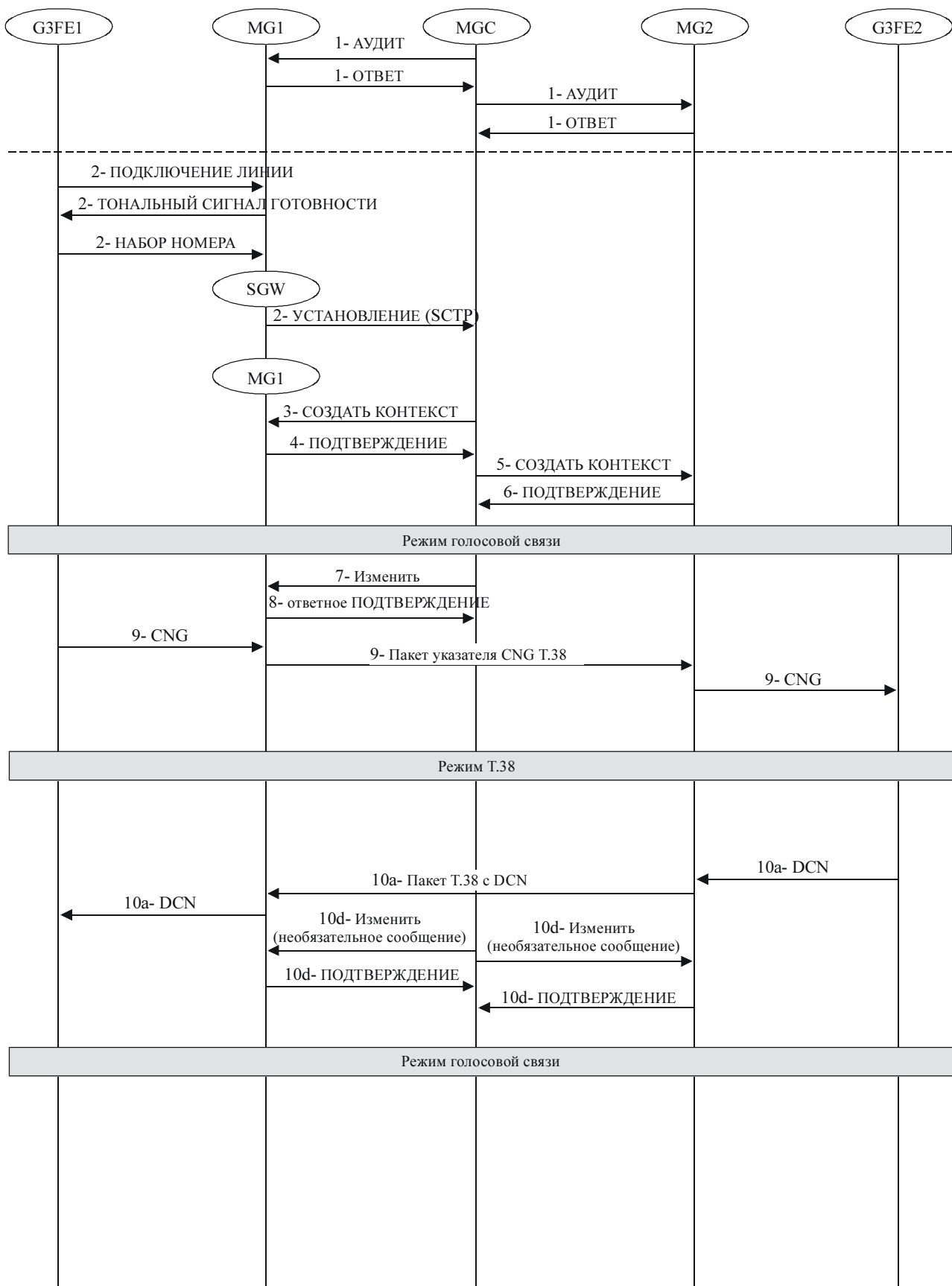
Рисунок III.3/T.38 – Установление соединения с переходом от голосовой к факсимильной связи с конечными точками H.248, которые поддерживают автономный метод перехода между VoIP и FoIP
