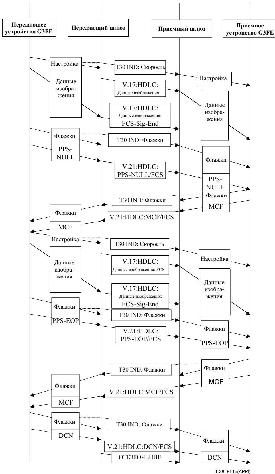
Рисунок I.1/T.38 – Два факсимильных устройства Группы 3, связь между которыми производится через шлюзы (лист 2 из 2)
