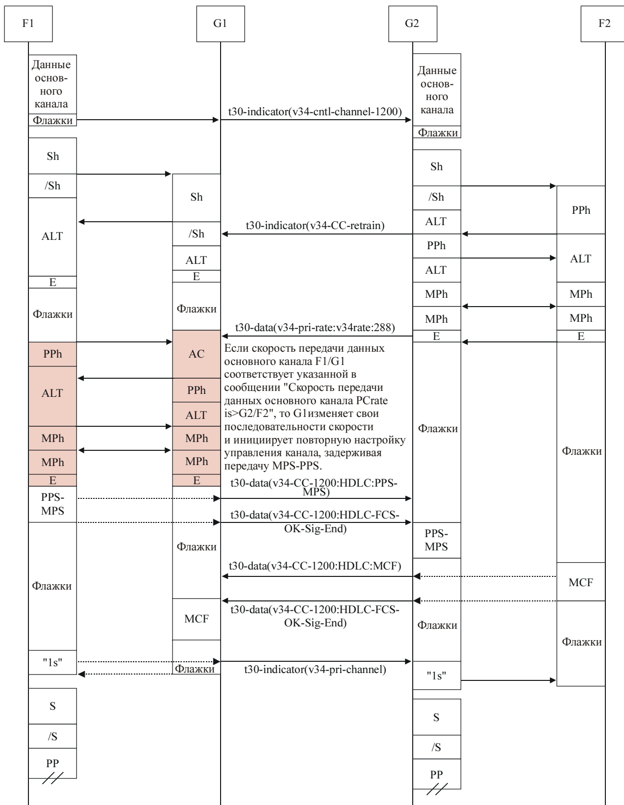
Рисунок IV.5/T.38 – Последовательность изменения скорости передачи данных, когда приемное устройство G3FE инициализирует повторную настройку
