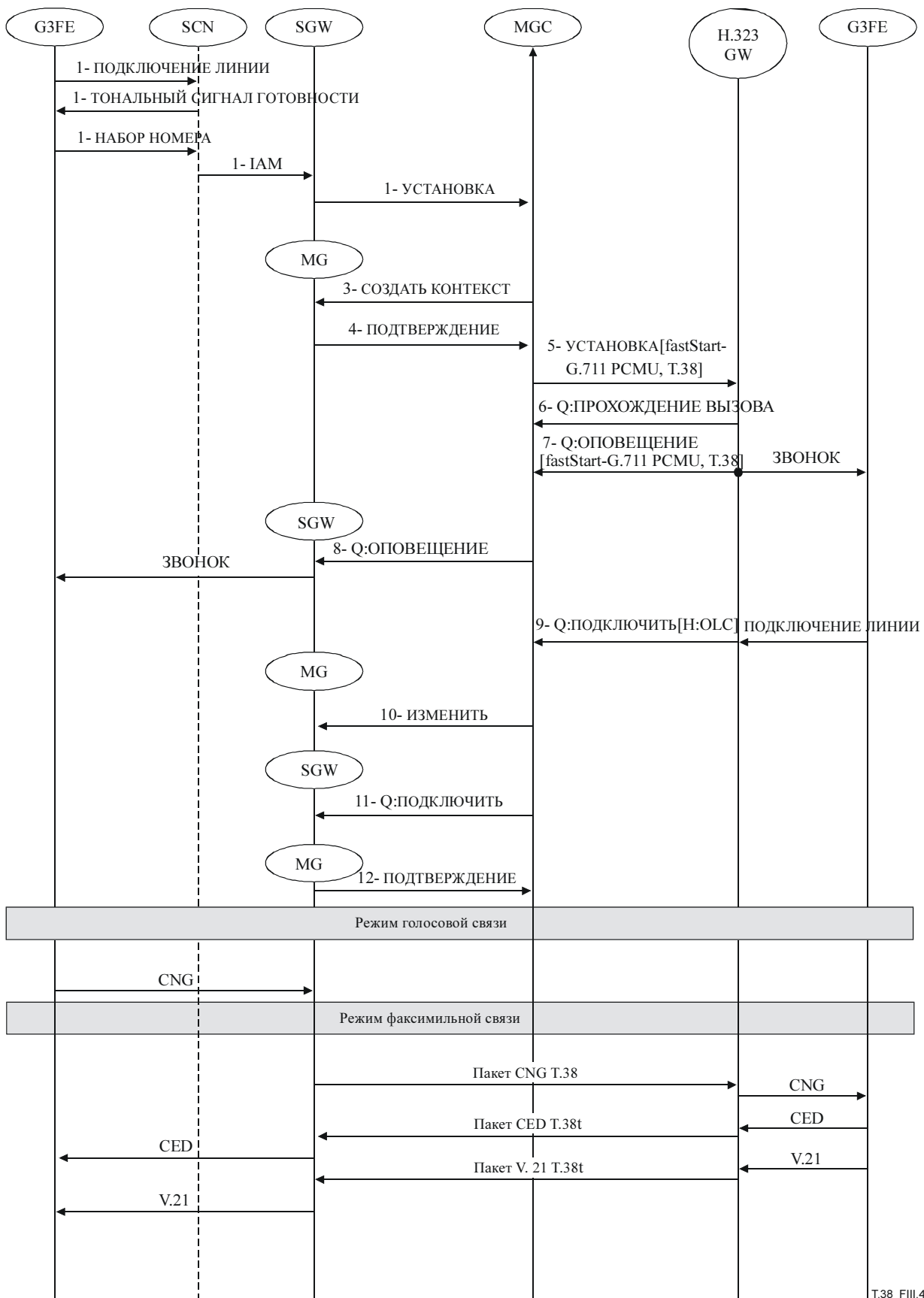
Рисунок III.4/T.38 – Установление соединения с переходом от голосовой к факсимильной связи между конечными точками H.248 и H.323, которые поддерживают автономный метод перехода согласно T.38 между VoIP и FoIP
