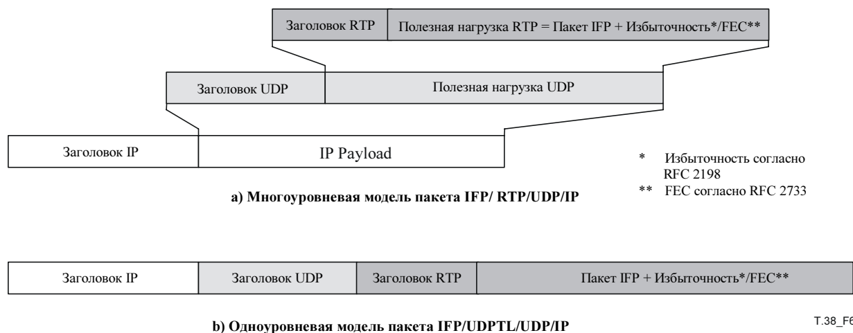
Рисунок 6/Т.38 – Структура пакета RTP/UDP/IP высокого уровня
