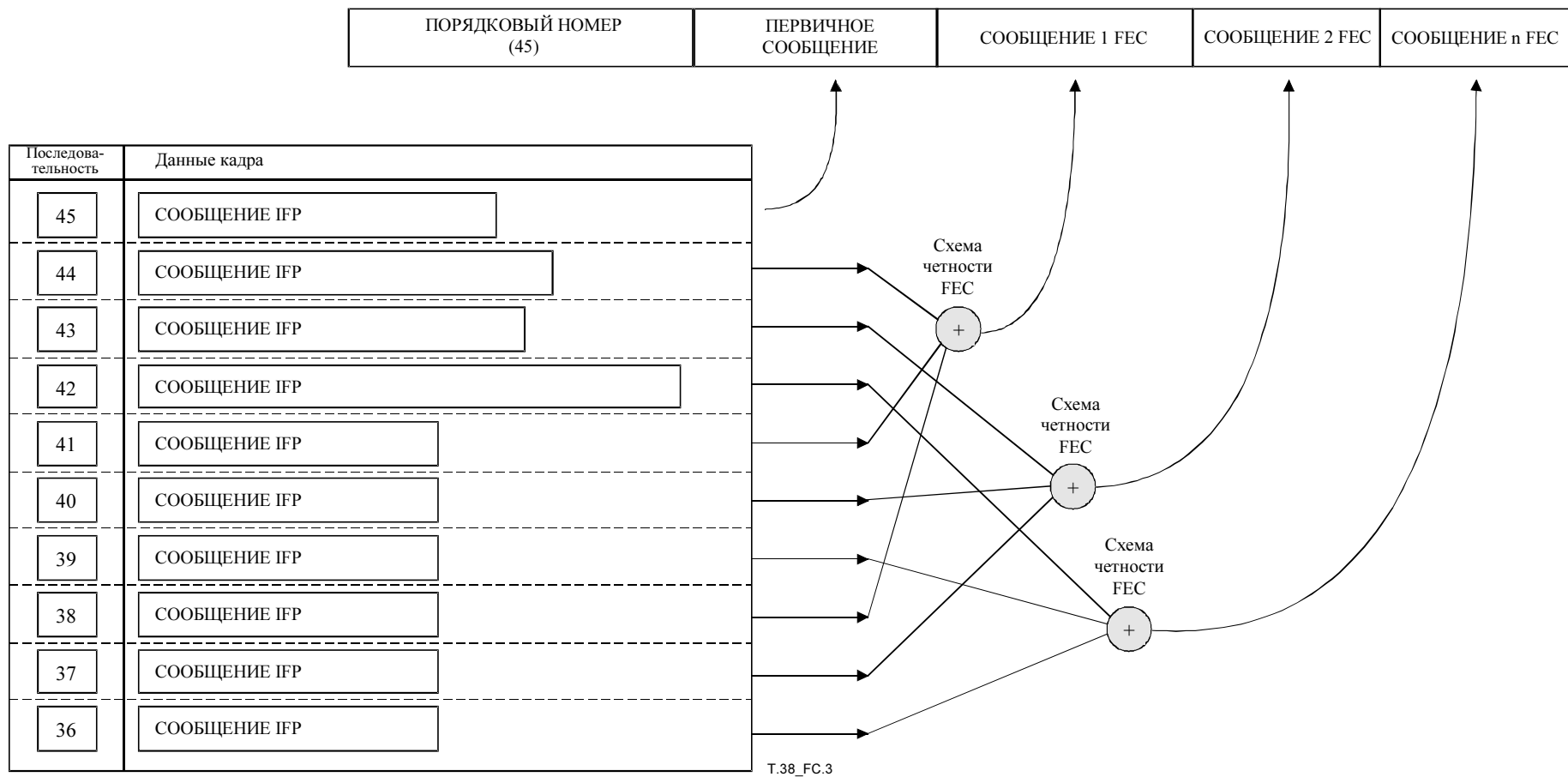
Рисунок С.3/Т.38 – Генерация множества сообщений FEC для защиты от пакета ошибок
