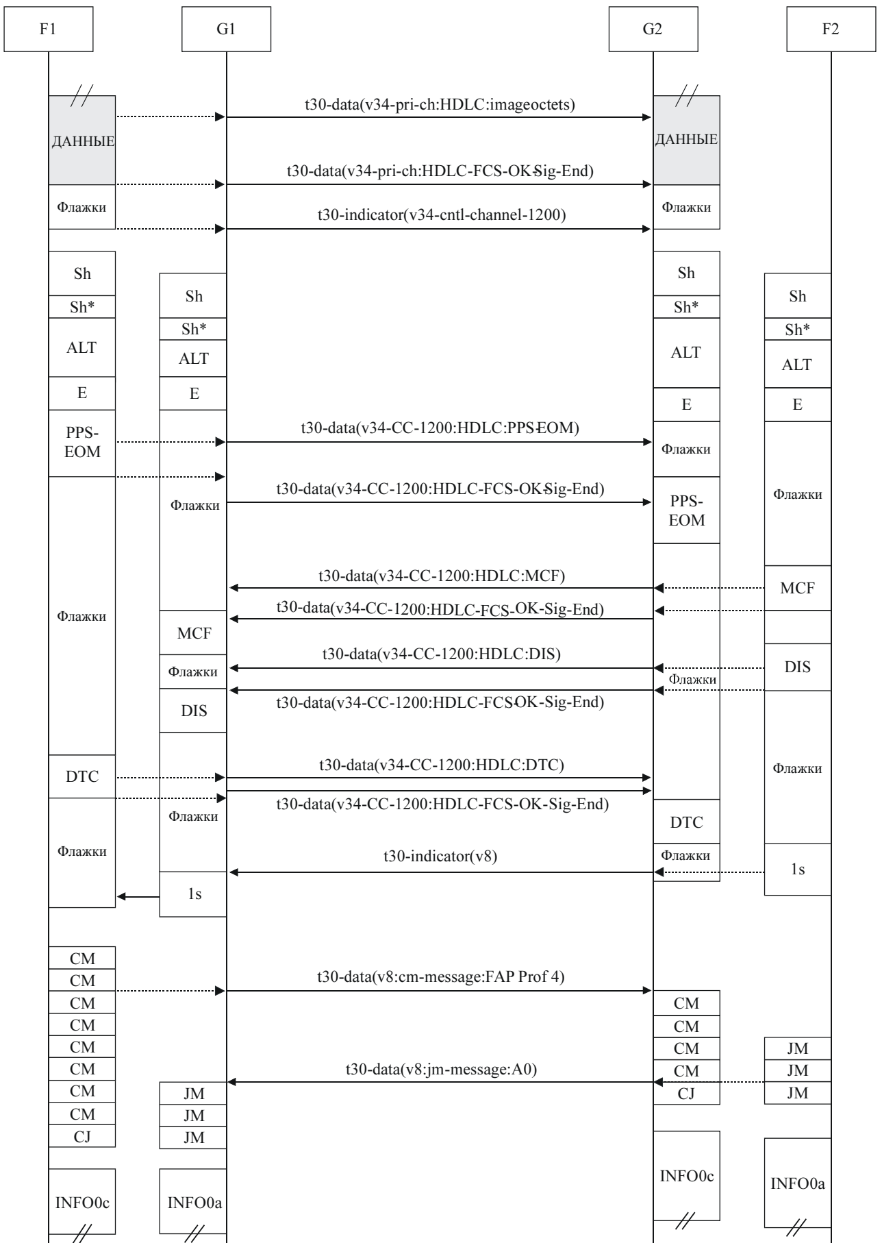
Рисунок IV.9/Т.38 – Опрос с последующим ответом
