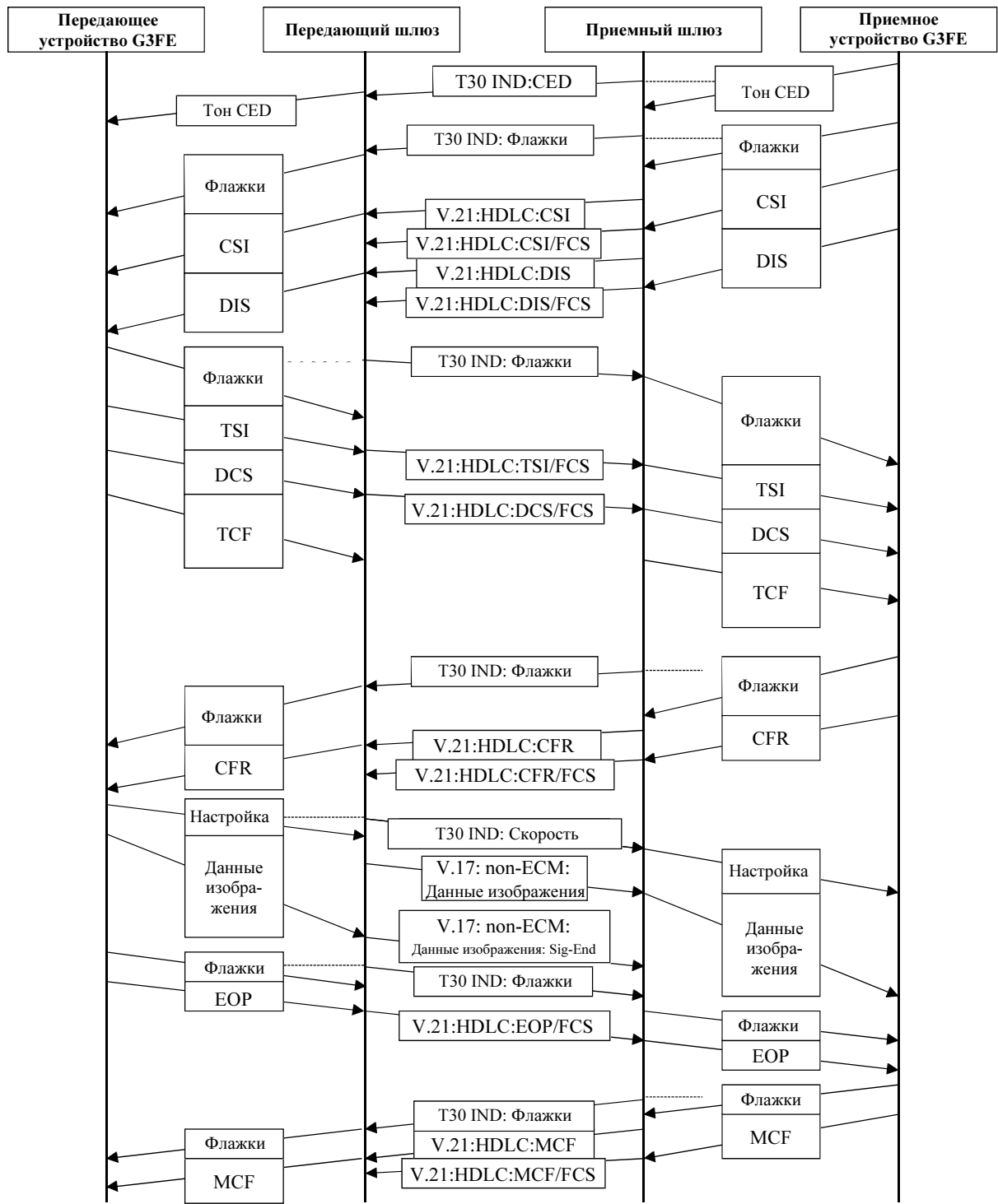
Рисунок I.3/Т.38 – Использование нескольких кадров на одну последовательность BCS
