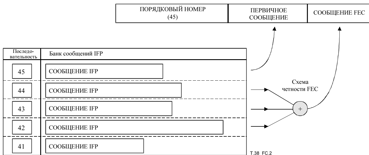
Рисунок С.2/Т.38 – Генерация и пакетирование одного кадра FEC четности
