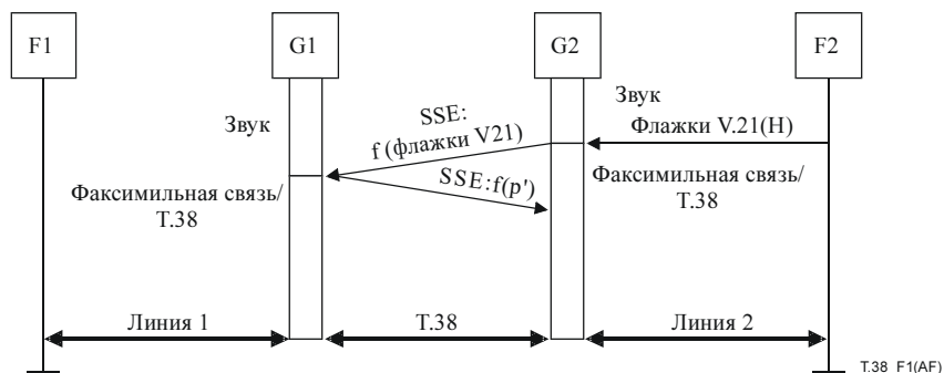
Рисунок F.1/T.38 – FoIP T.38 (переход от MoIP к факсимильной передаче T.30)
