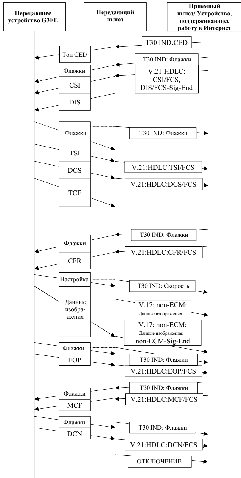
Рисунок I.2/Т.38 – Обычное факсимильное устройство и устройство, поддерживающее работу в интернете
