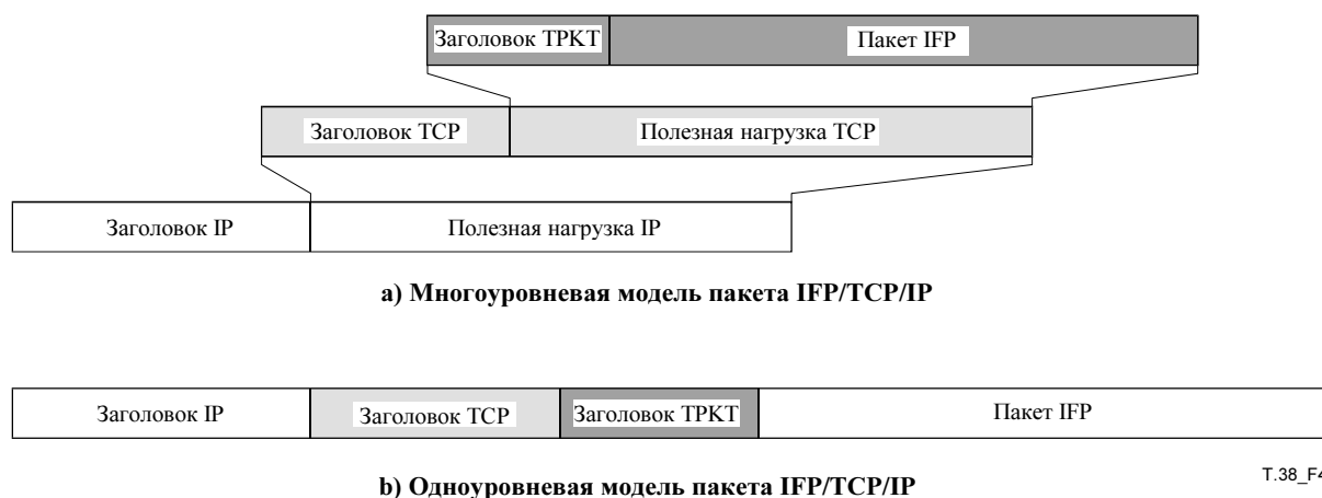
Рисунок 4/Т.38 – Структура пакета TCP/ТРКТ/IP высокого уровня
