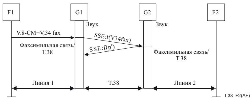
Рисунок F.2/T.38 – FoIP T.38 (переход от MoIP к факсимильной передаче V.34)
