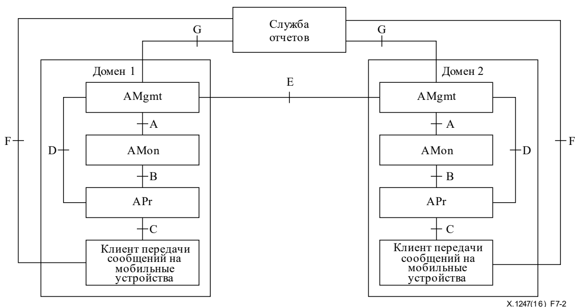
Рисунок 7-2 – Эталонная модель
