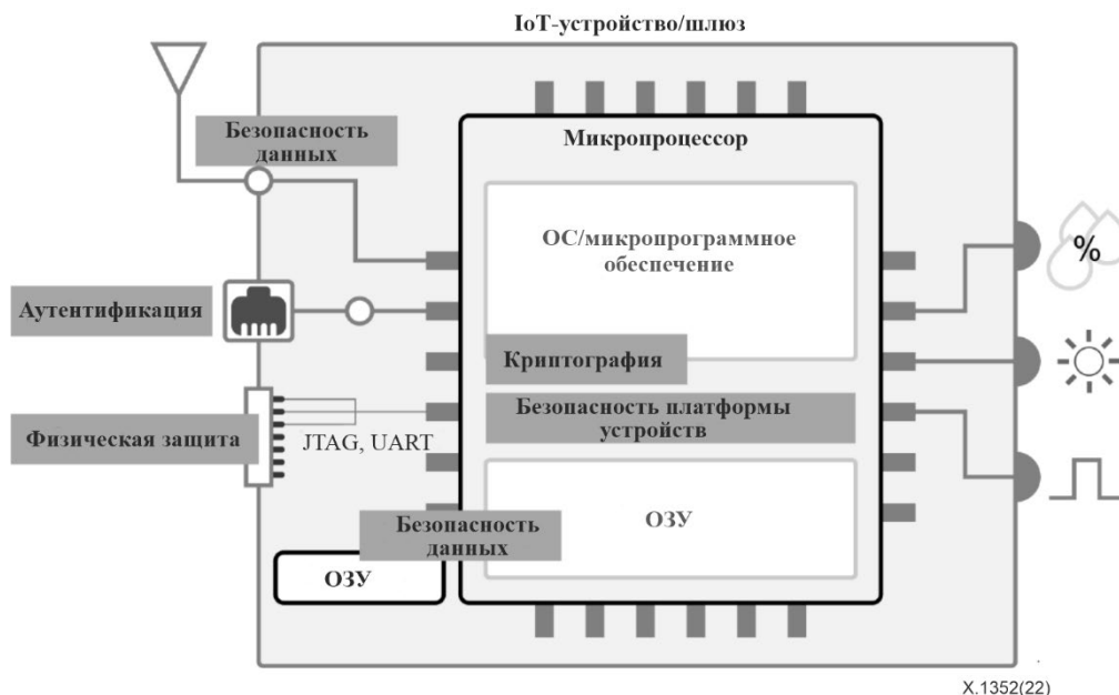
Рисунок 2 – Пример применения средств безопасности в устройствах и шлюзах IoT
