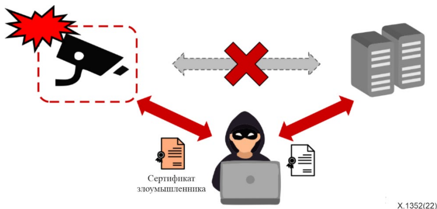
Рисунок II.1 – Пример аутентификации
