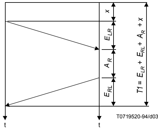
FIGURA 3/X.224
