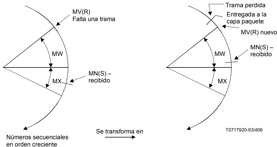
FIGURA 2-4/X.25 Detección de pérdida de tramas multienlace
